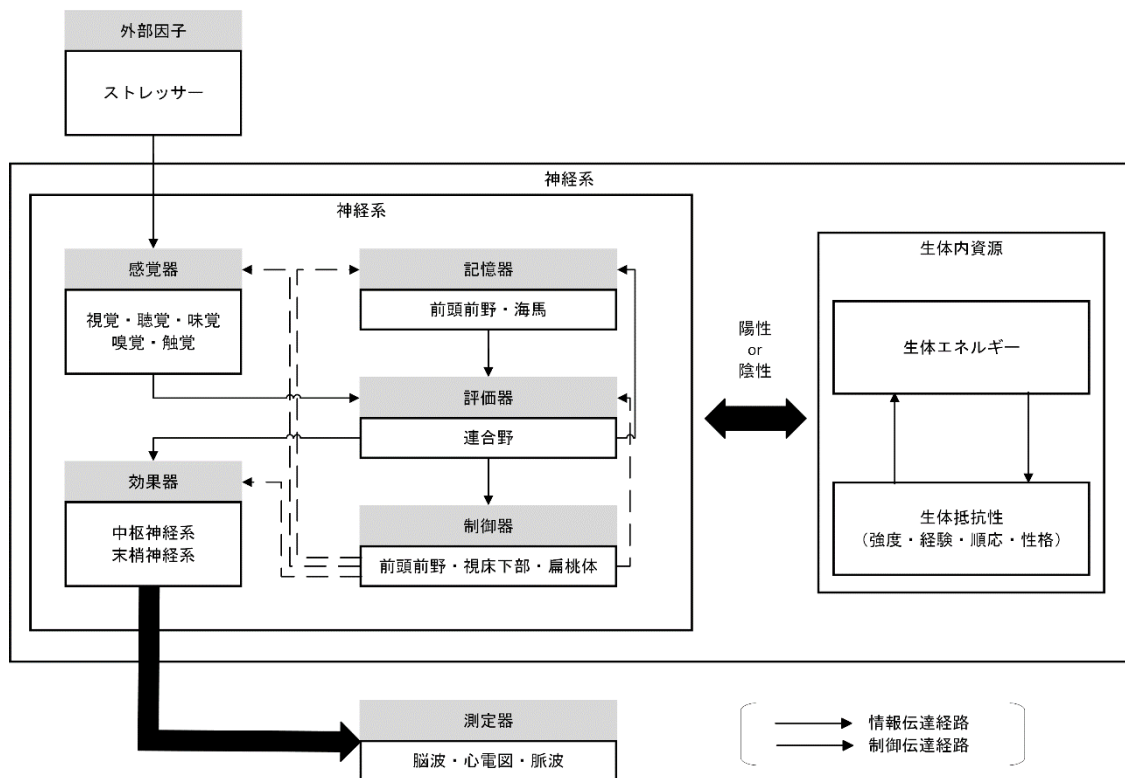
図 7.3：ストレスに関連した生体情報処理システム
