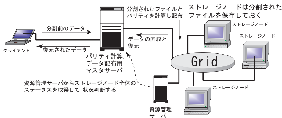
図 3.1: システム構成図 (各サービスが独立している状態)
