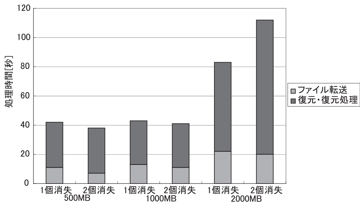
図 5.9: 縮退運転時の性能
