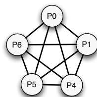
図 2.4: Neko Topology
