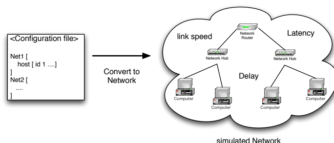
図 2.5: SSFNet
