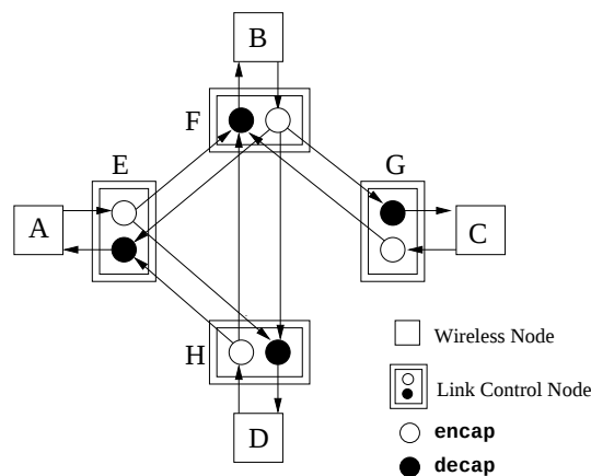
図 4.5: カプセル化
