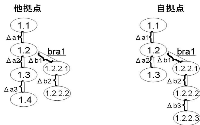
図 5.1: 実行前
