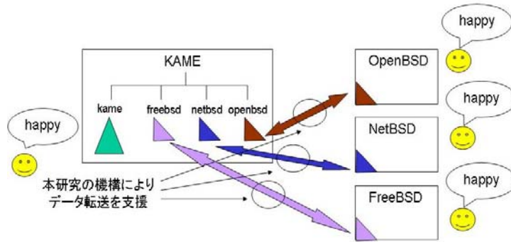
図 6.2: KAME
