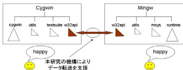
図 6.1: Cygwin
