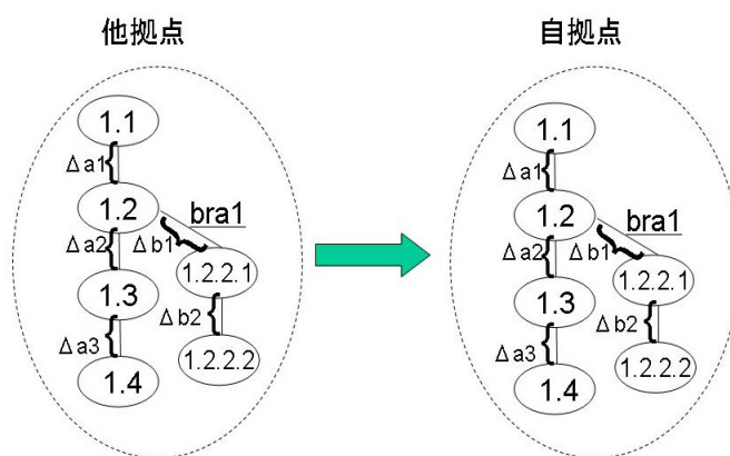
図 5.2: 実行後
