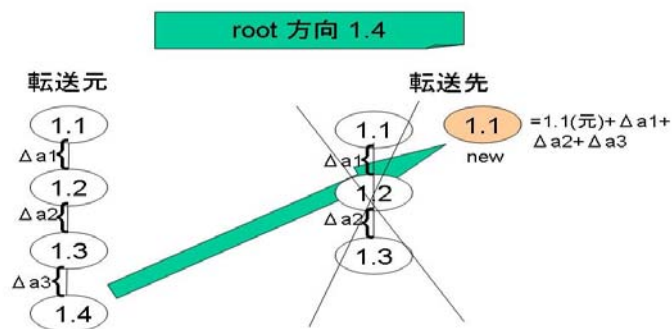
図 3.13: root 上書き
