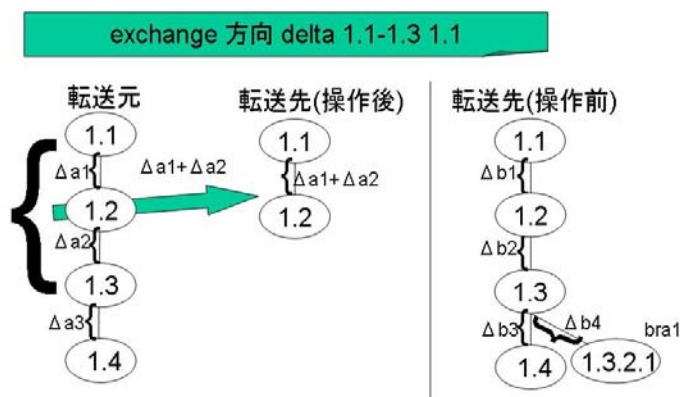
図 3.18: exchange 上書き
