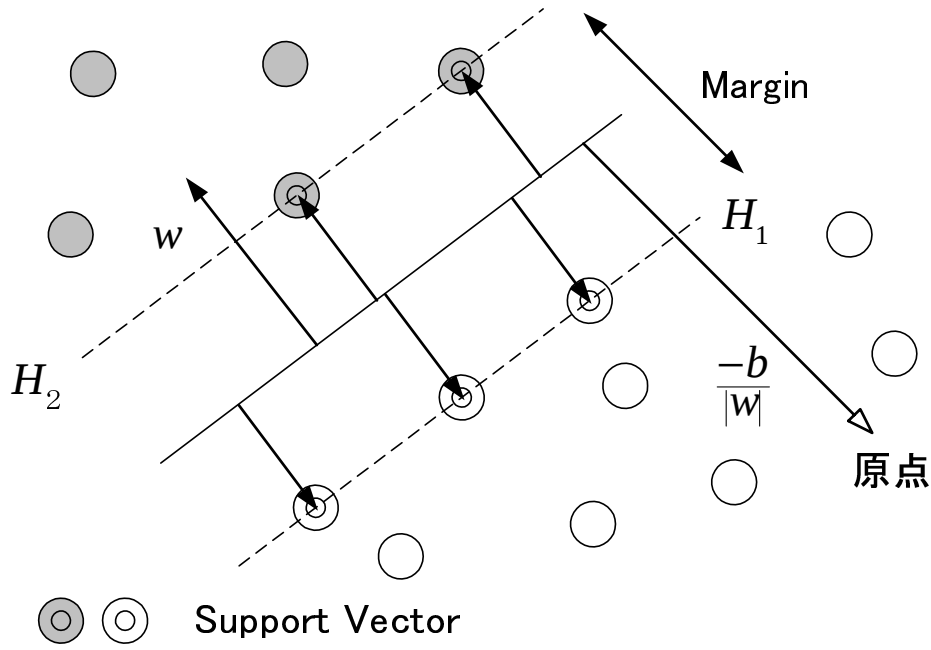
図 4.1: SVM 概要
