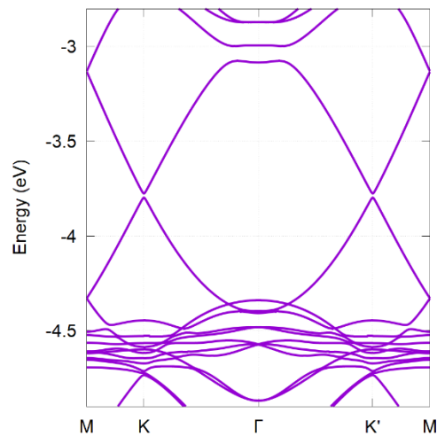
図 2. グラフェン/MoS2 のバンド構造
