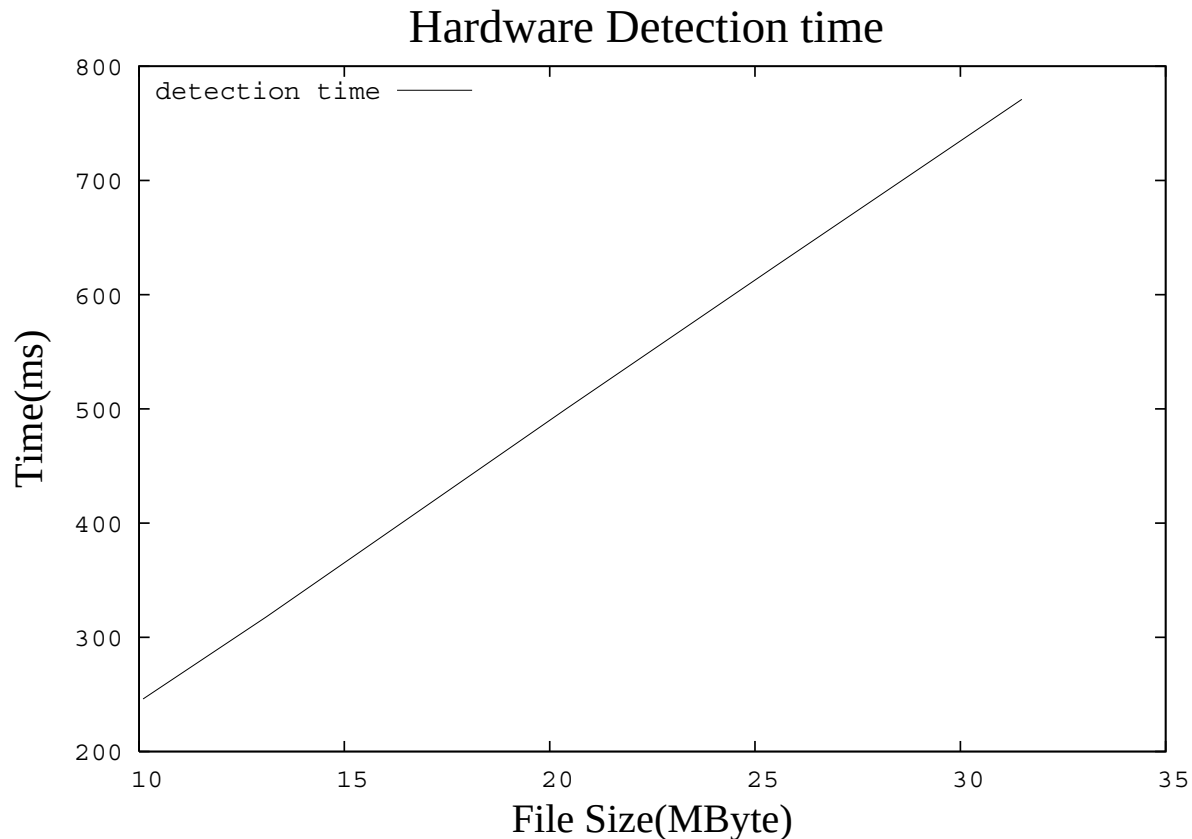
図 4.3: 検出時間の推移
