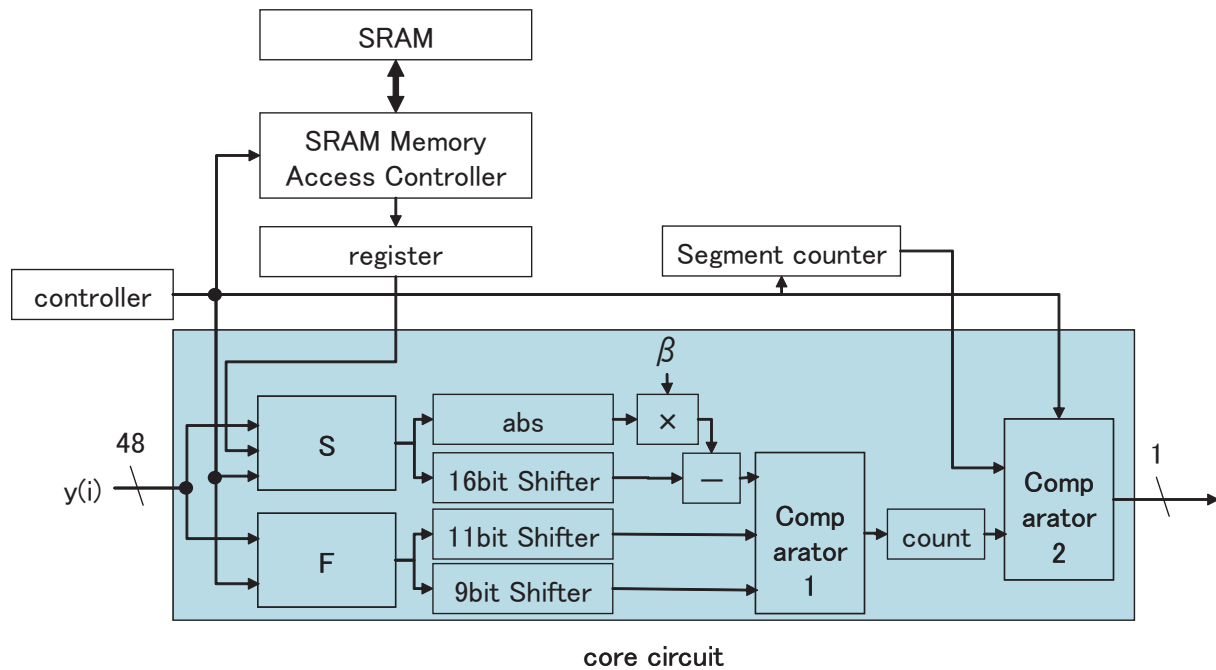
図 3.12: 1つの透かし検出回路
