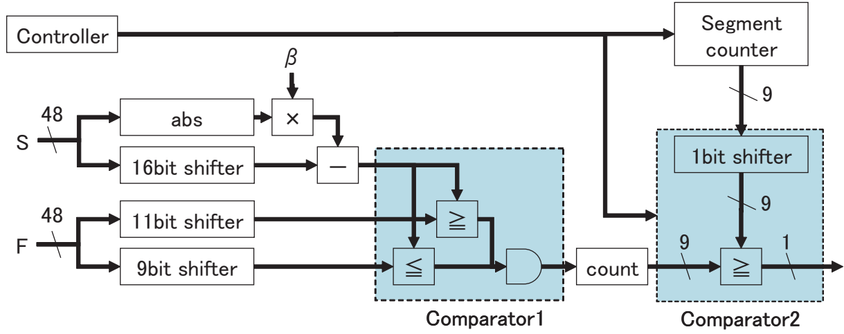
図 3.11: 比較演算ユニット
