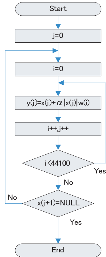
図 2.2: 透かし埋め込み
