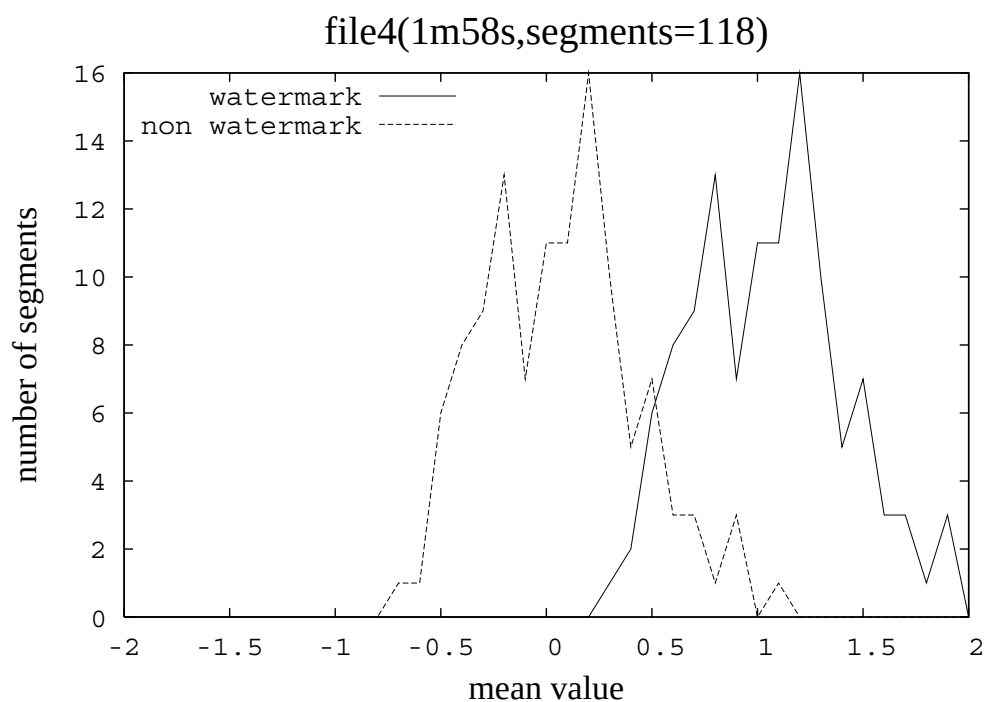
図 3.6: ファイル 4 の r の度数分布
