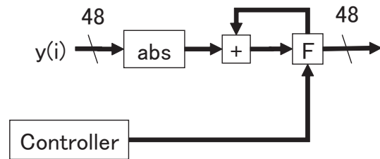
図 3.10: F 演算ユニット
