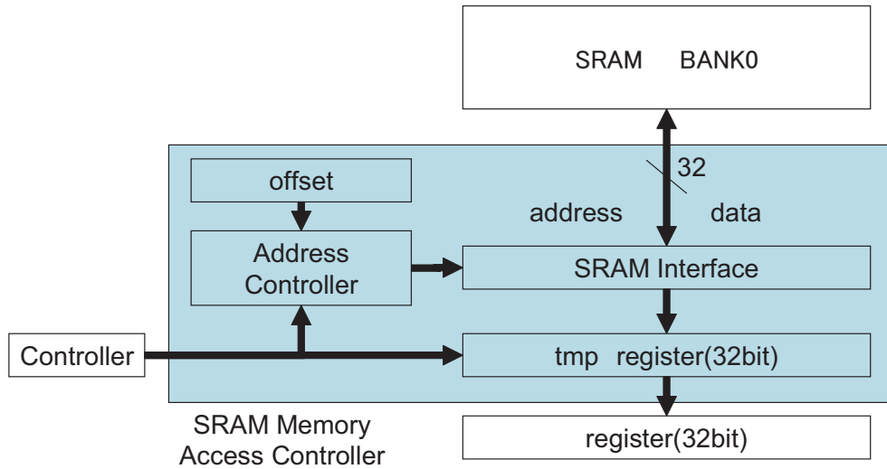
図 3.8: 透かしデータ転送ユニット
