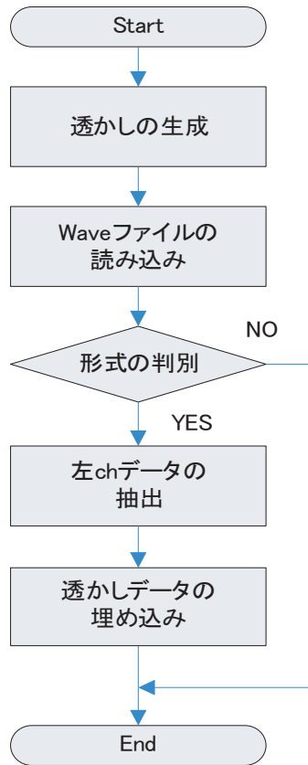
図 2.1: 埋め込みフローチャート
