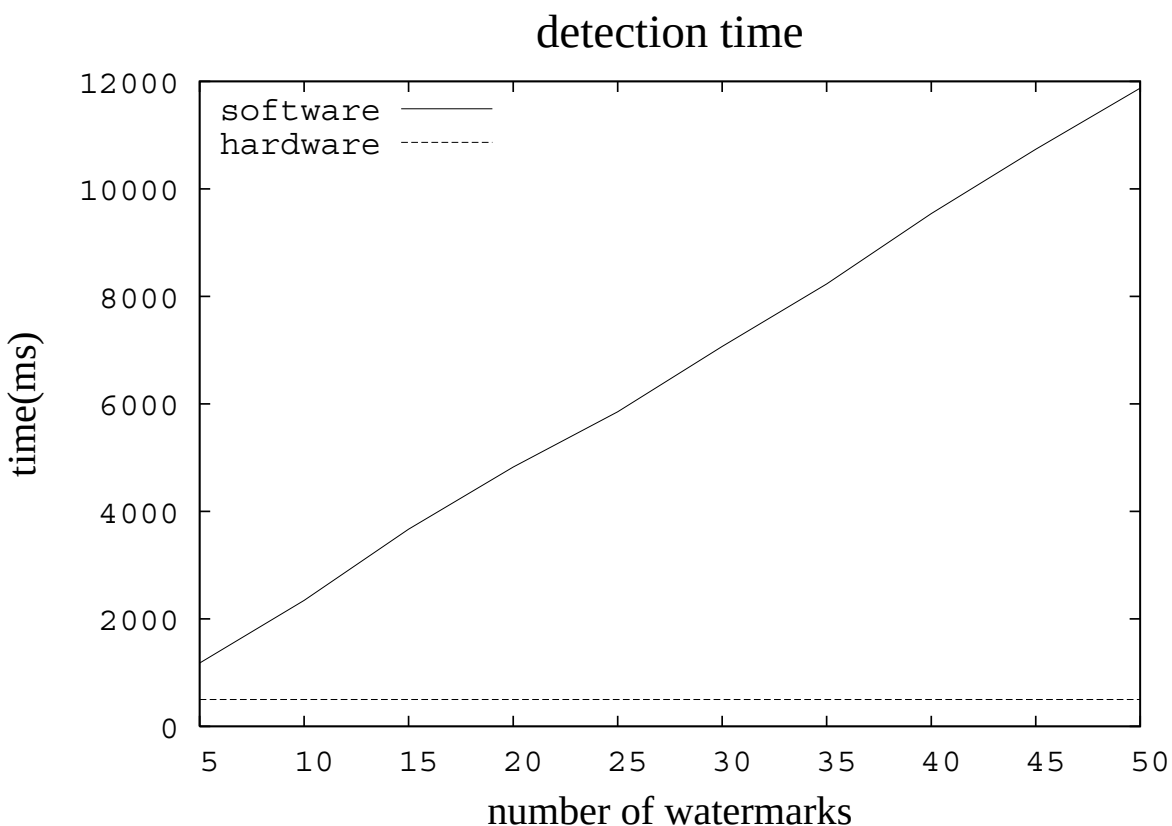
図 4.2: 検出時間の比較
