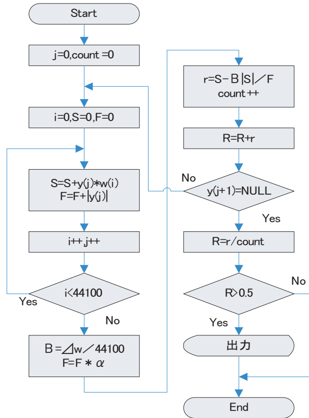
図 2.4: 透かしの検出
