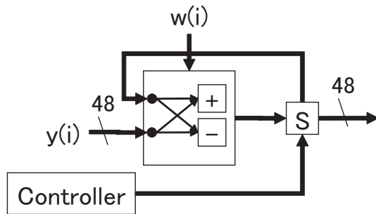
図 3.8: 透かしデータ転送ユニット
