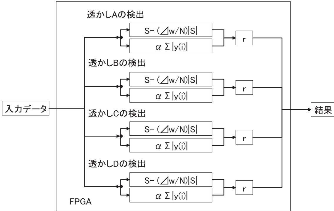
図 3.1: 検出回路の並列化
