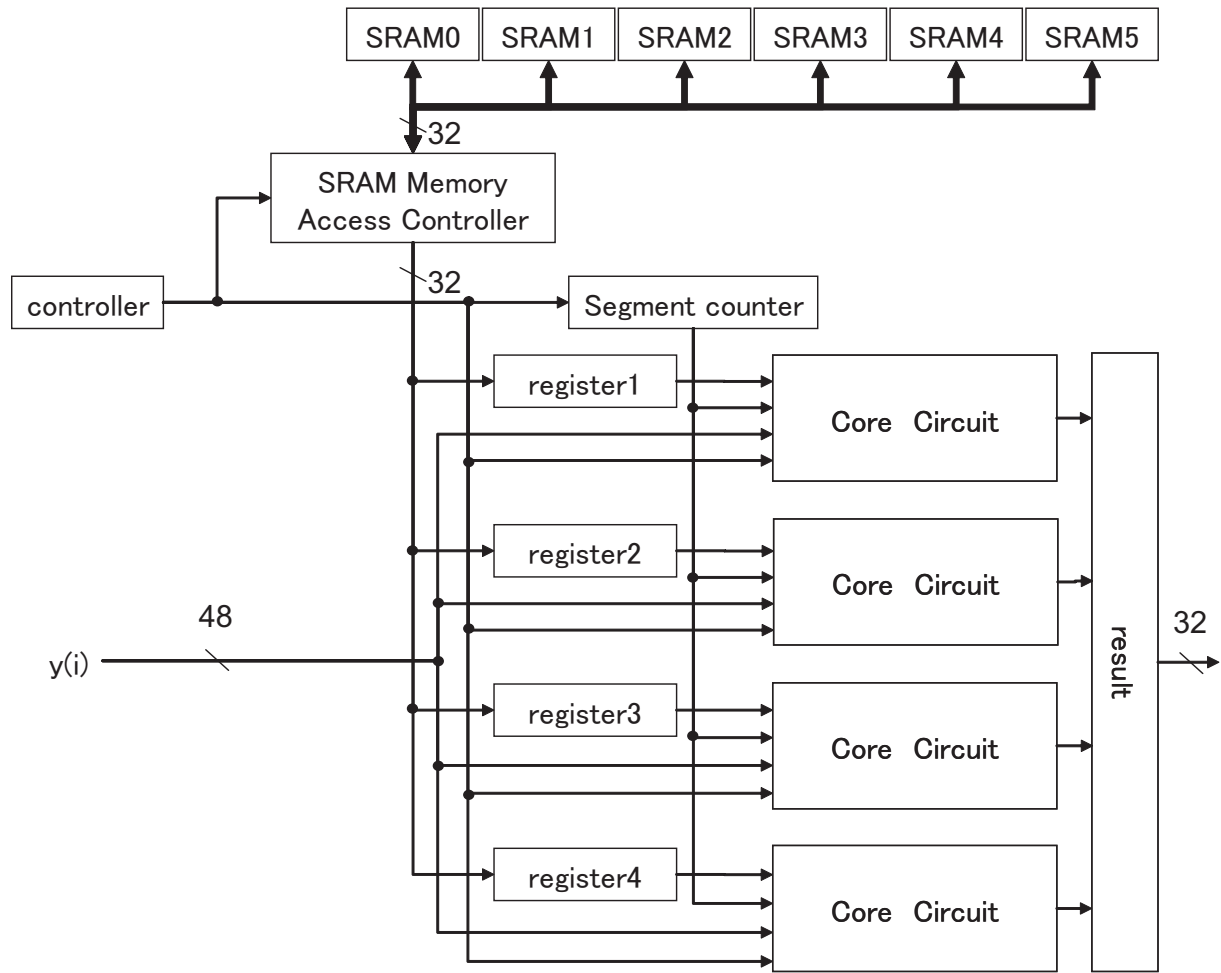
図 3.13: 複数の透かし検出回路
