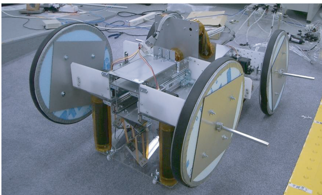
図 2.1: 探索支援型ロボット JAI-Rover-I
