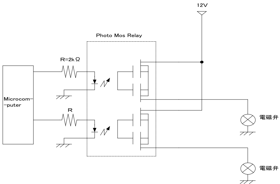
图 5.7: 回路構成例
