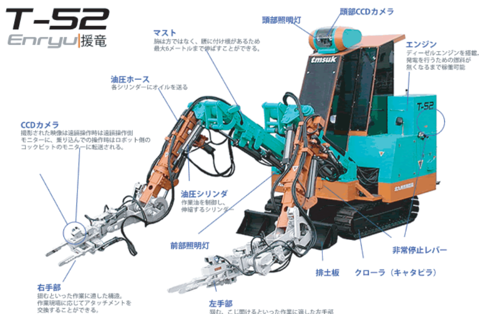
図 2.2: 障害物除去支援型ロボット 援龍 T-52
