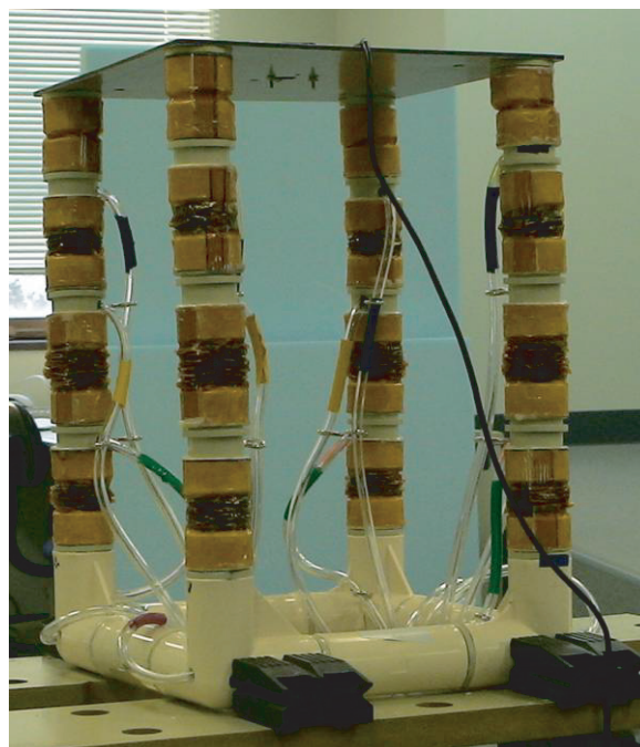
図 5.2: 本研究室で開発した FSB-module( l=200 [mm])
