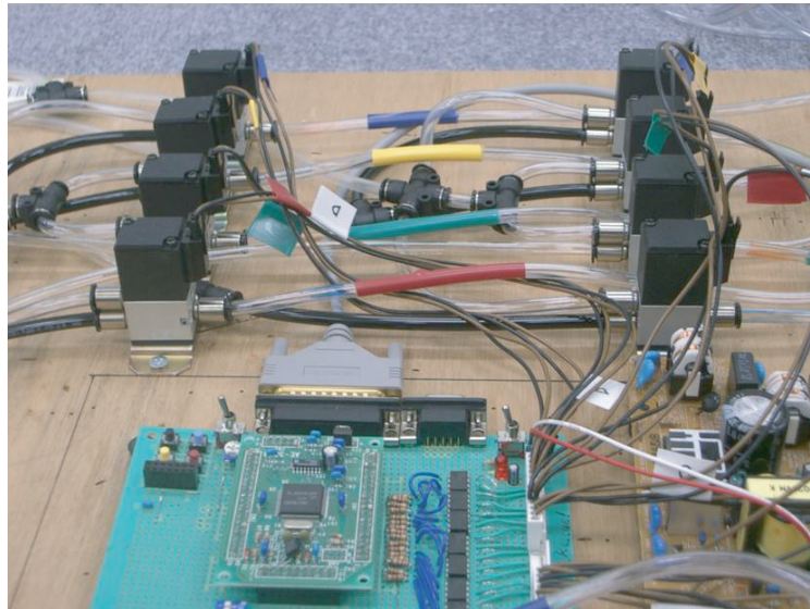
图 5.8: 回路構成:实物写真
