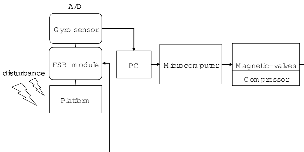
図 5.3: フィードバック制御システム
