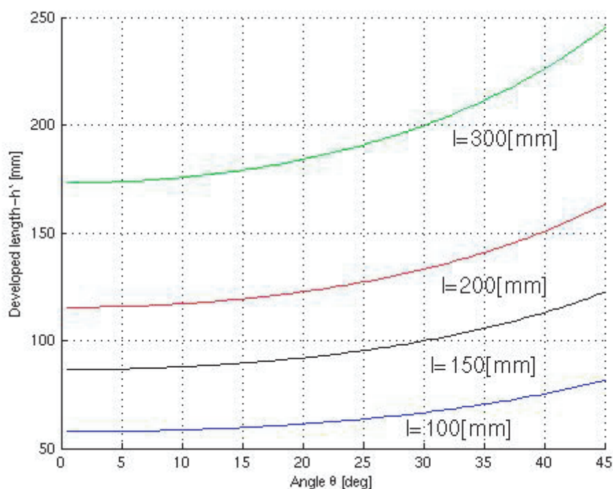
図 5.1: 各一辺 l での展開幅 h'
