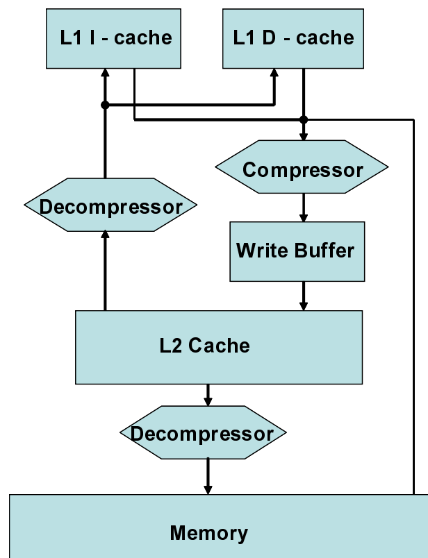
図 3.1: メモリ階層
