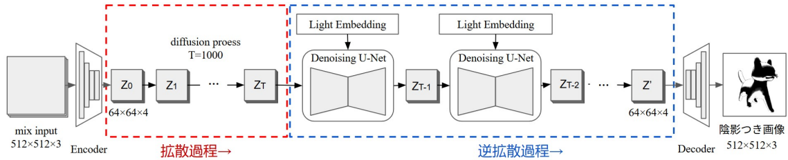
図 4.6 : Diffusion モジュールの構造
