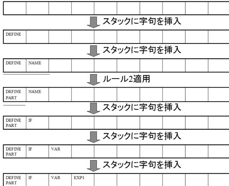
図 5.4: スタック内の動作 1
