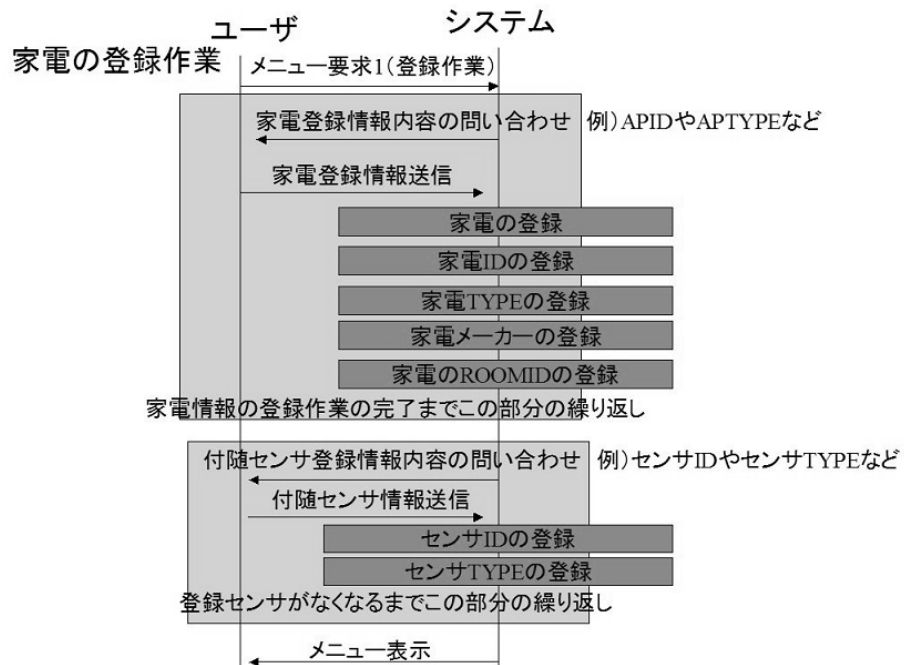
図 6.3: 家電の登録
