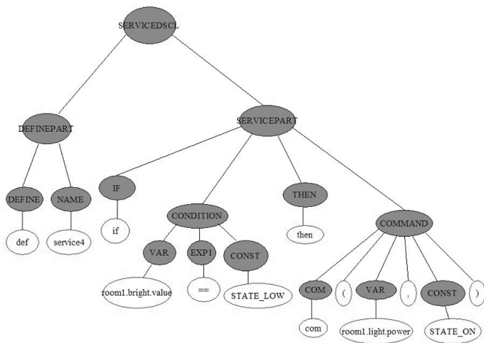
図 7.4: 構文木 4
