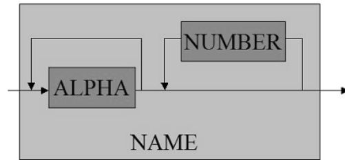
図 A.3: 名前
