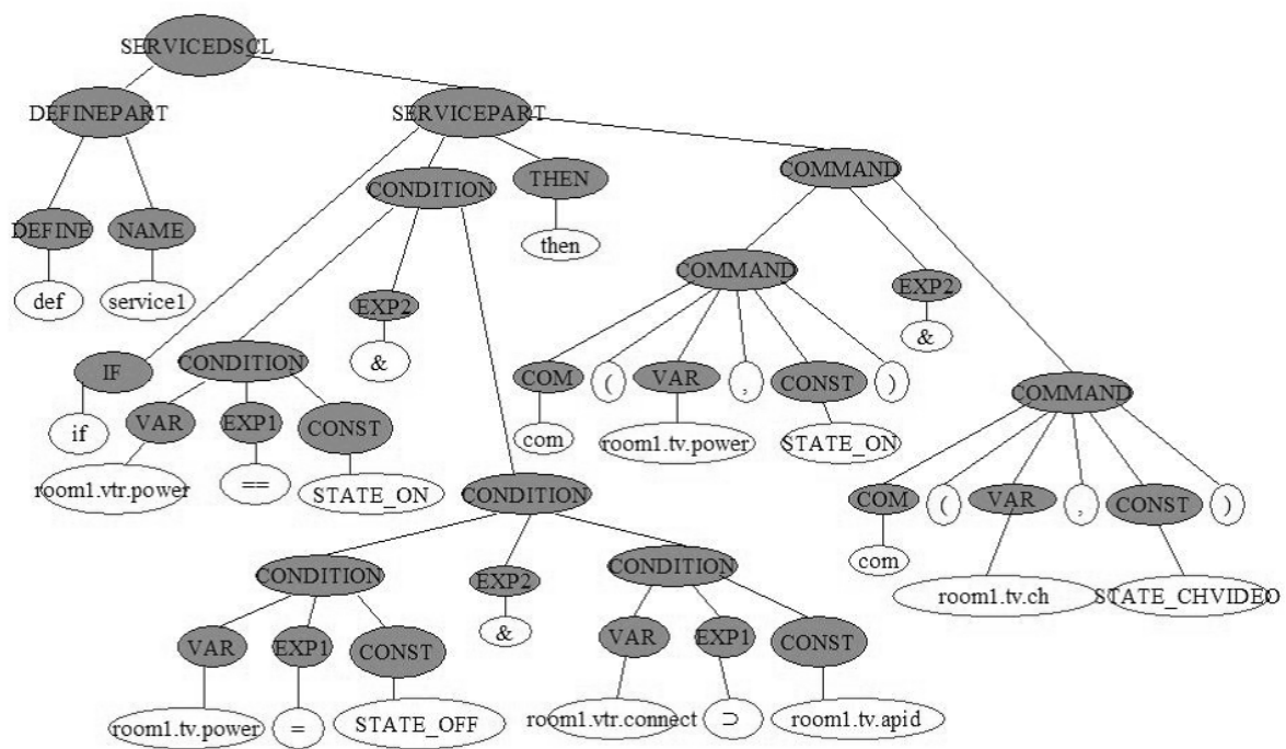
図 7.1: 構文木 1
