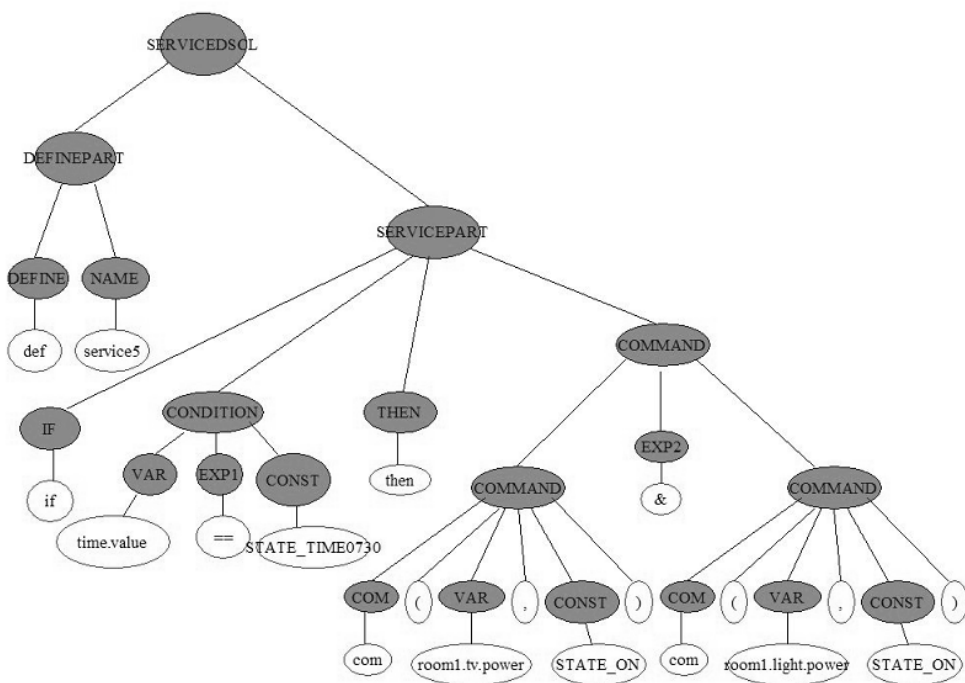
図 7.5: 構文木 5
