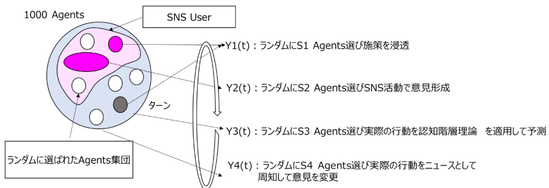
図 20 エージェントシミュレーションの実行フロー
