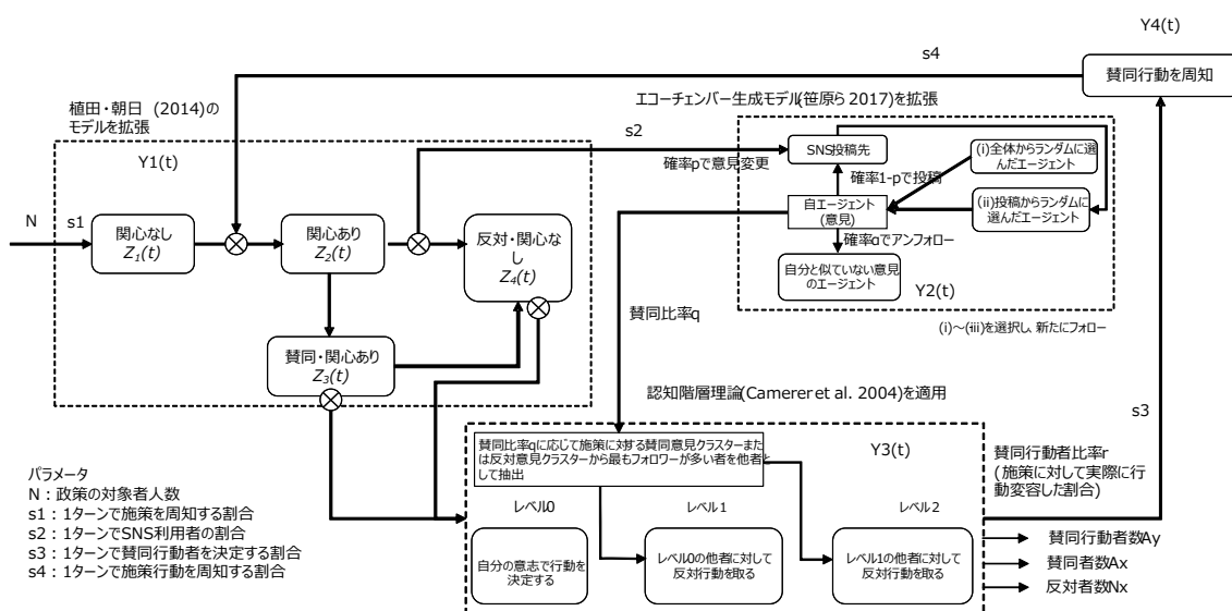
図 18 提案モデルの全体像
