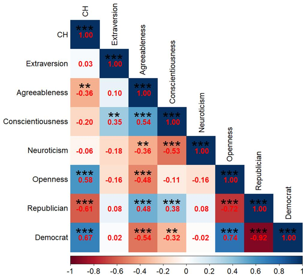
図 53 政党支持率、他者に対する思考に関する平均値 (CH)、Big Five パーソナリティ、それぞれの間の相関 (カラーマップは相関 (-1.0 から 1.0) の大きさを表し、青が 1.0 で赤が-1.0、色の濃さが値の大きさに対応する。***、**、*は 1%、5%、10%の有意水準で有意差があることを表す)
