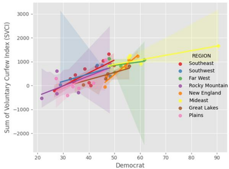
図 51 全米 8 地域の SVCI と 2016 年大統領選挙における民主党への投票率との関連性 (縦軸：外出自粛指数の総和 SVCI、横軸：民主党への投票率 (%)、半透明部分： 95%信頼区間、点は回帰プロット、直線は回帰直線を表す)
