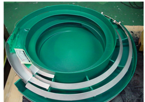
図-1 パーツフィーダボウル内面塗装施工
