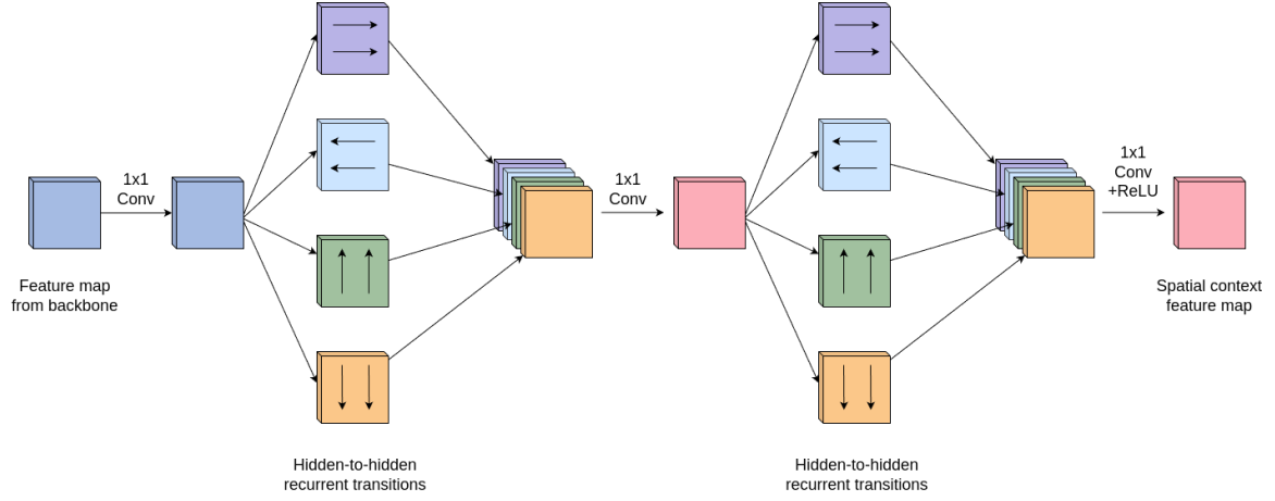
Fig. 7. Spatial RNN module
