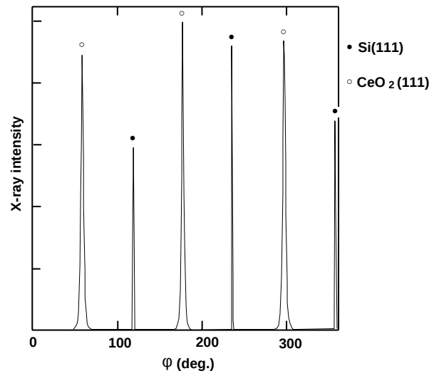
図 1: \text{CeO}_2 エピ膜の \phi スキャン
