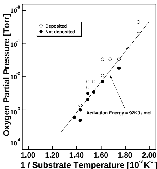
図 1: 膜堆積に必要な酸素分圧と成膜温度の関係
