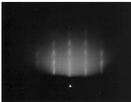
図 1: \text{CeO}_2[112] の RHEED 像
