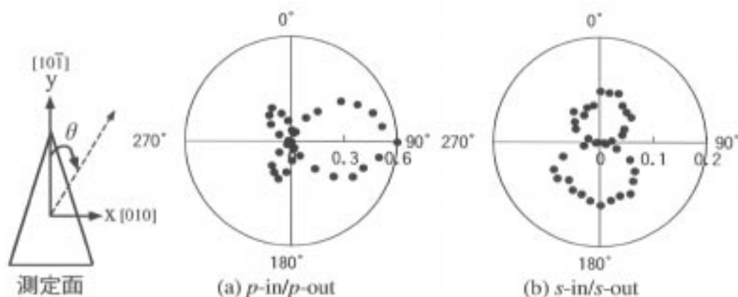
図 1: アナターゼ型 \text{TiO}_2 (101) の SH 光強度方位角依存性
