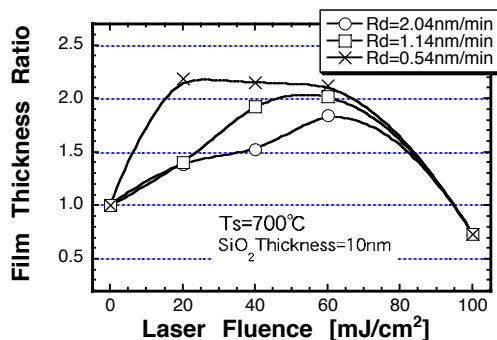
図 1: 各堆積速度における膜厚比のフルーエンス依存性
