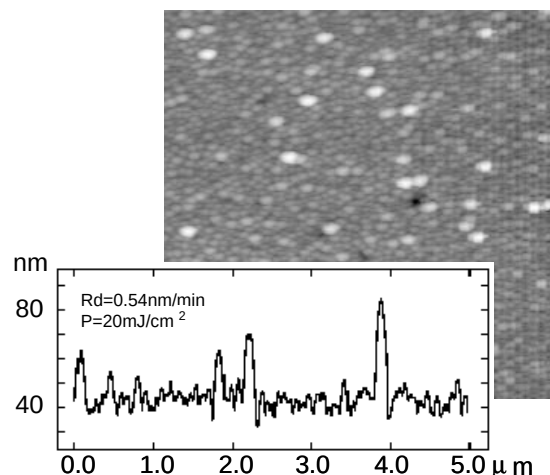
図 2: Si 凝集粒子の AFM 像及び断面プロファイル
