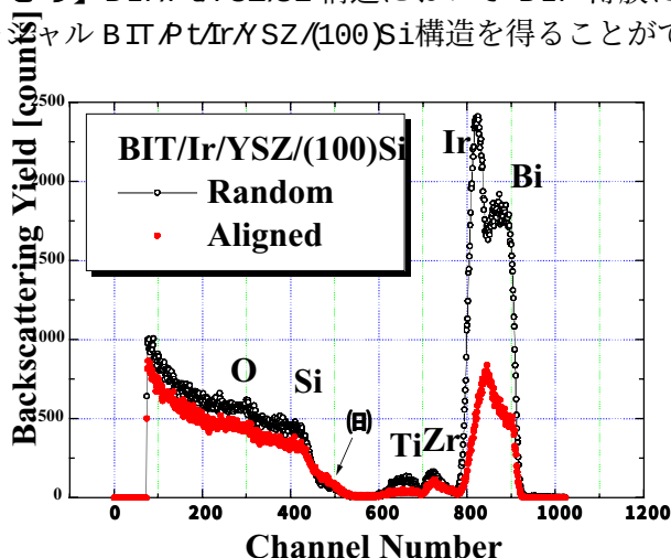
図 1 BIT/Ir/YSZ/(100)Si 積層構造の RBS スペクトル
