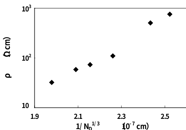
図 1 \text{As}_{\text{Ga}} の平均距離に対する比抵抗の変化
