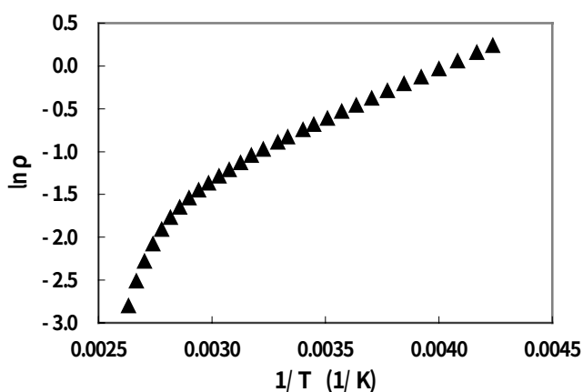
図 2 超薄膜 LT-GaAs の比抵抗の温度による変化
