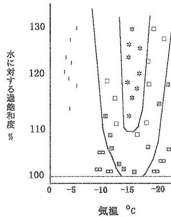
図 2: 中谷ダイヤグラム
