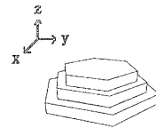
図 3: 結晶と層の関係
