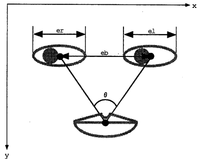
図 18: 顔部品大きさ・位置関係
