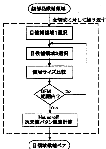
図 19: 目領域候補ペア抽出処理の流れ
