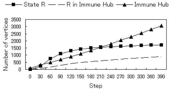
図 20 免疫状態の頂点数 (ハブ免疫化 20%)
