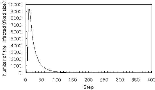
図 7 固定規模における感染数の変化
