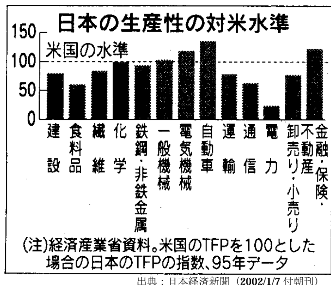
図 5-2 日本の産業の対米 TFP 水準
