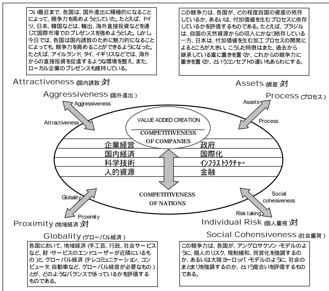
図 3-4 WCY の「4つの競争環境」コンセプト
