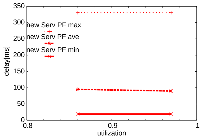
図 A.3: 提案手法 PF クラスのフレーム遅延
