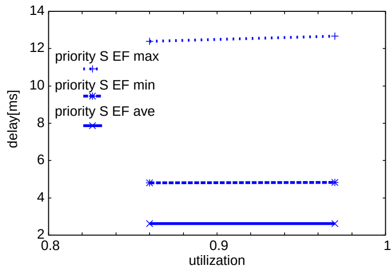
図 A.2: 優先スケジューリング EF クラスのフレーム遅延
