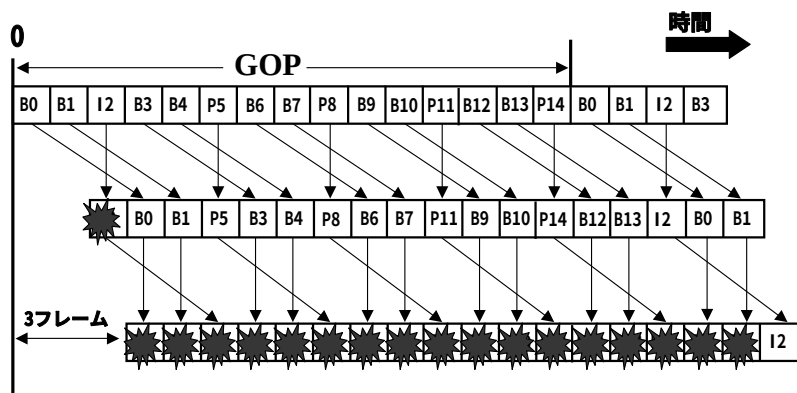
図 4.5: I ピクチャエラー時の影響範囲
