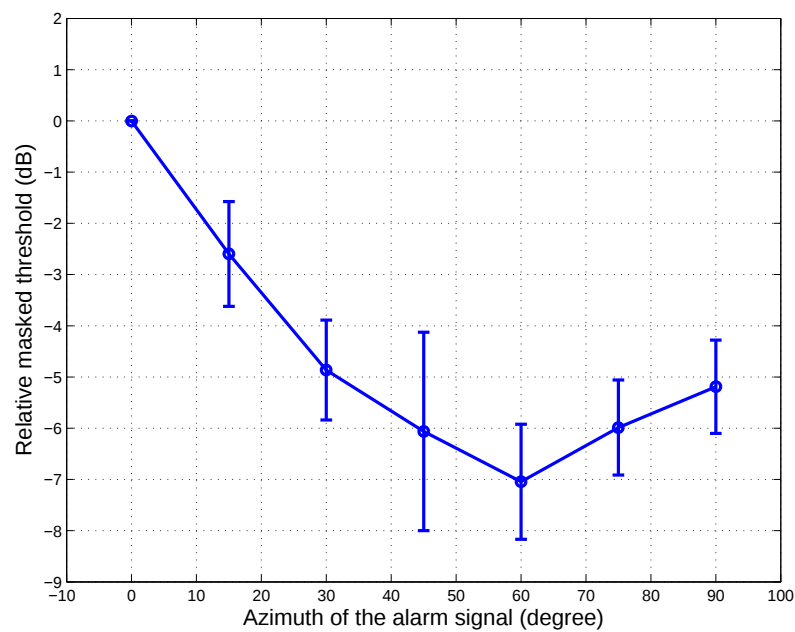
図 4.1: 1.0 kHz の S_m N_0 条件の報知音のマスキング閾値: 被験者 5 名に対する平均
