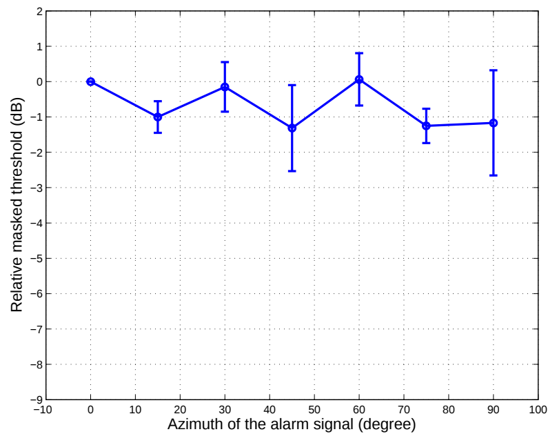
図 4.2: 4.0 kHz の S_m N_0 条件の報知音のマスキング閾値: 被験者 8 名に対する平均
