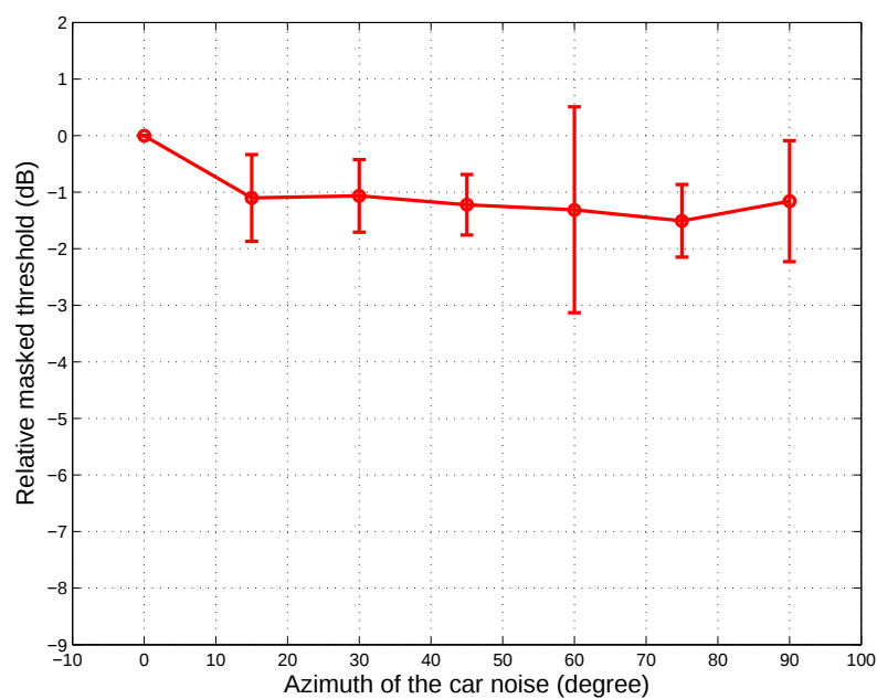
図 7.2: S_0N_m 条件における走行雑音下のパルス音のマスキング閾値: 被験者 4 名に対する平均
