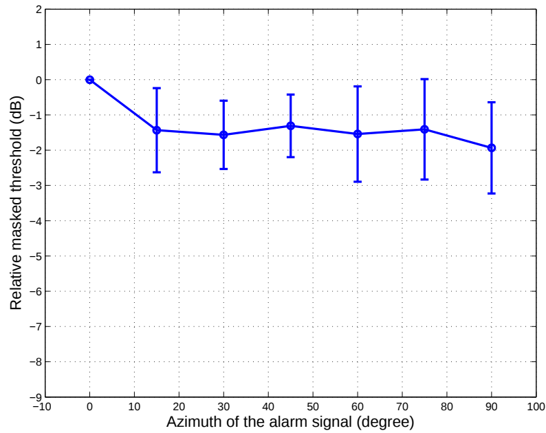
図 7.1: S_0N_m 条件における走行雑音下のパルス音のマスキング閾値: 被験者 6 名に対する平均
