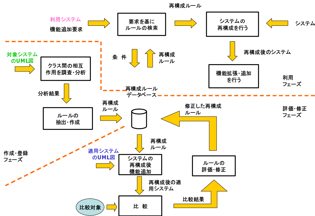
図 3.1: 再構成規則の全体図
