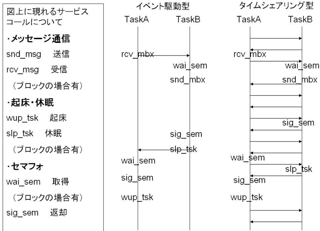
図 3.2 イベント駆動型とタイムシェアリング型のディスパッチタイミングの違い
