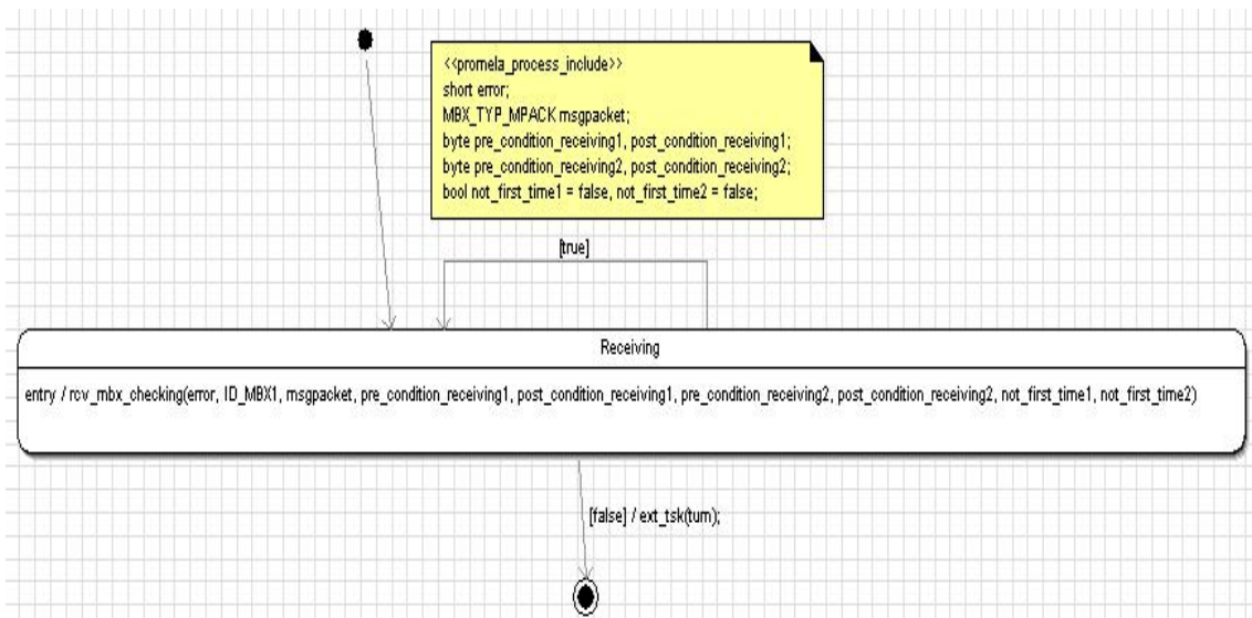
図 4.2 検証用外部モデル 1 (受信タスクのステートマシン図)
