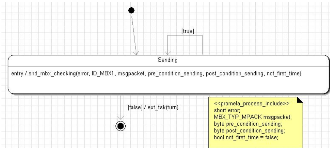
図 4.2 検証用外部モデル 1 (送信タスクのステートマシン図)
