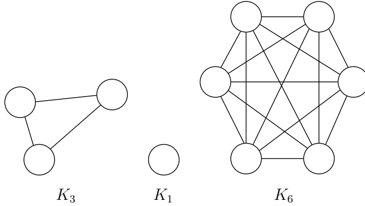
図 2.3: 完全グラフ
