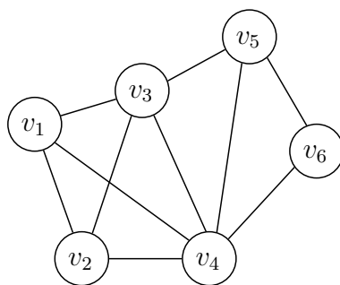
図 2.4: グラフ G
