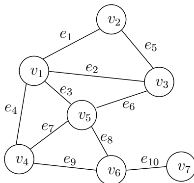
図 2.1: グラフ
