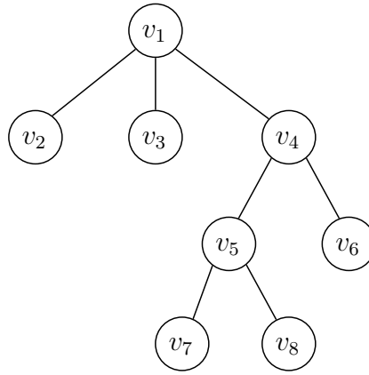
図 2.6: 根付き木
