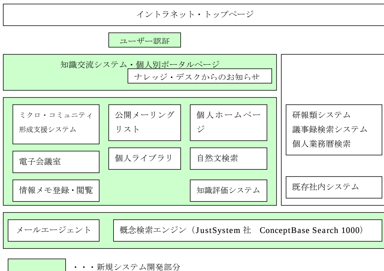
図 3.6.1 知識交流システム構成図
