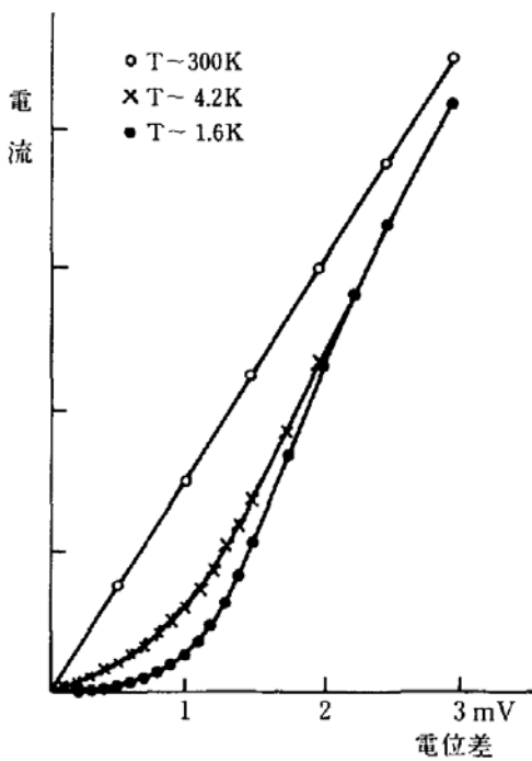
第13図 アルミ-酸化アルミ-鉛の電圧-電流特性 (このデータはギャーバーによってとられたもの)
