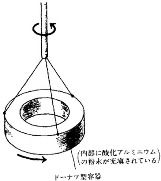
第 11 図 液体ヘリウムの 永久流
