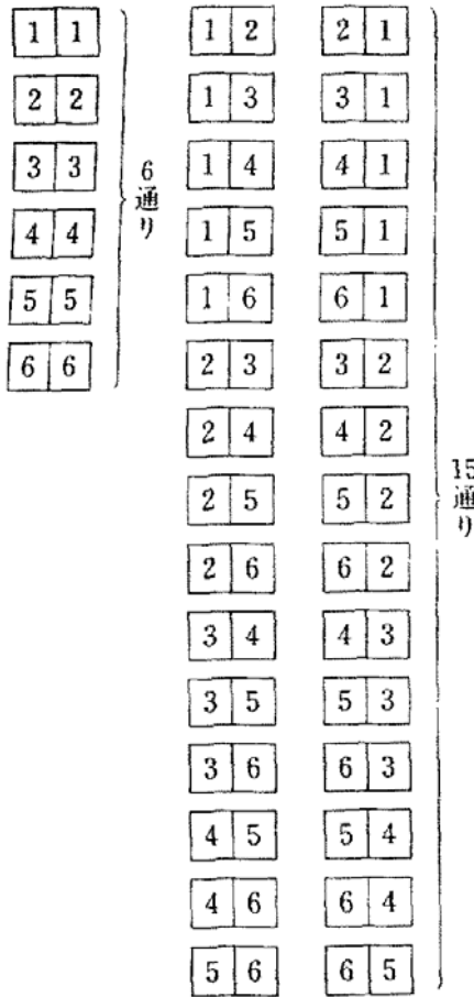
第 13 図 状態の数
