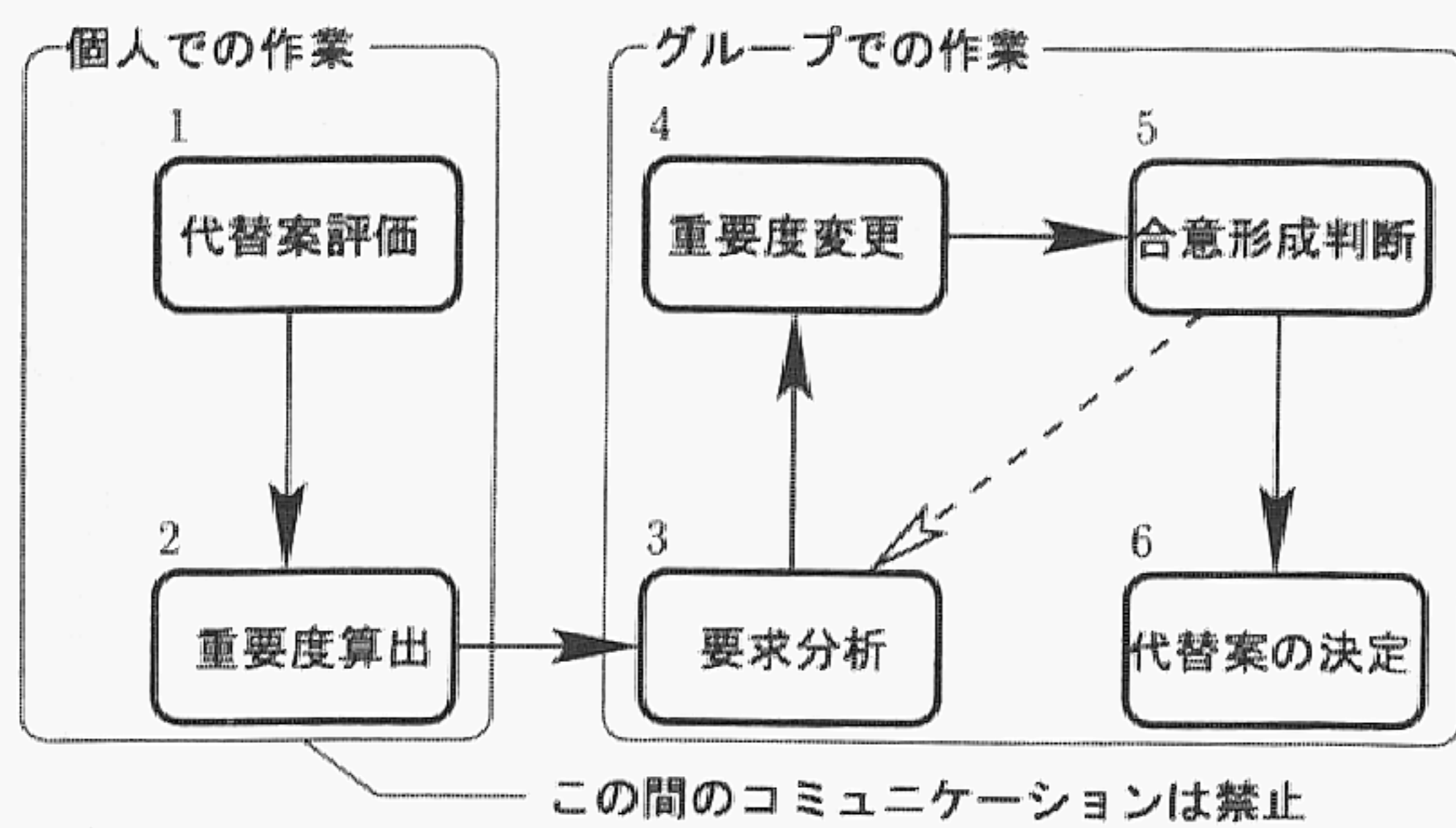
図2 実験で用いたグループ意思決定支援プロセス
