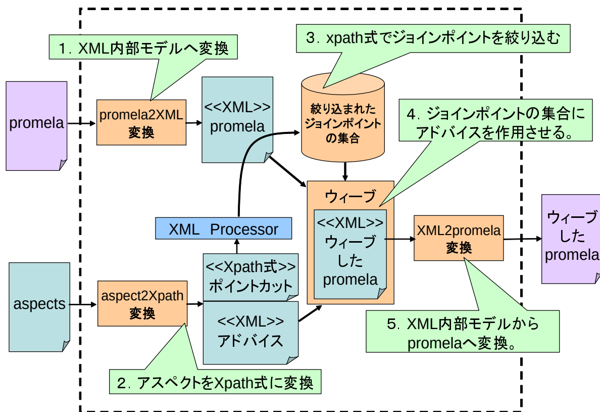
図 6.1: 言語処理系の全体図
