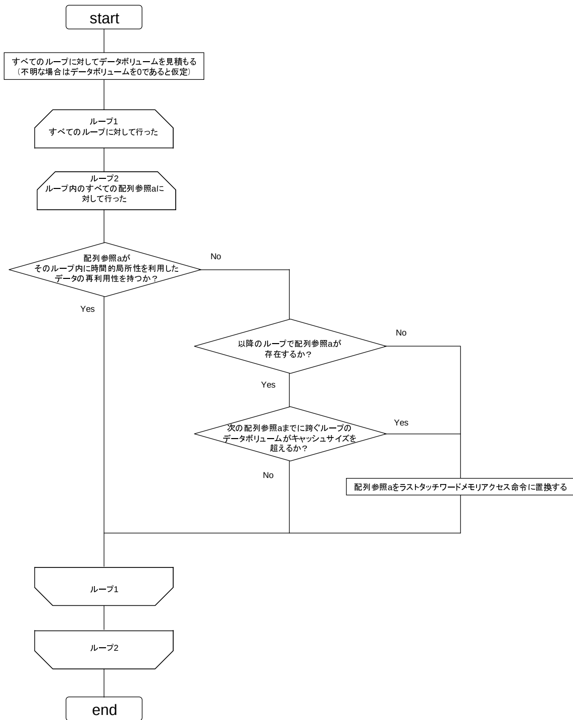
図 4.2: ラストタッチメモリアクセス命令への置換アルゴリズム
