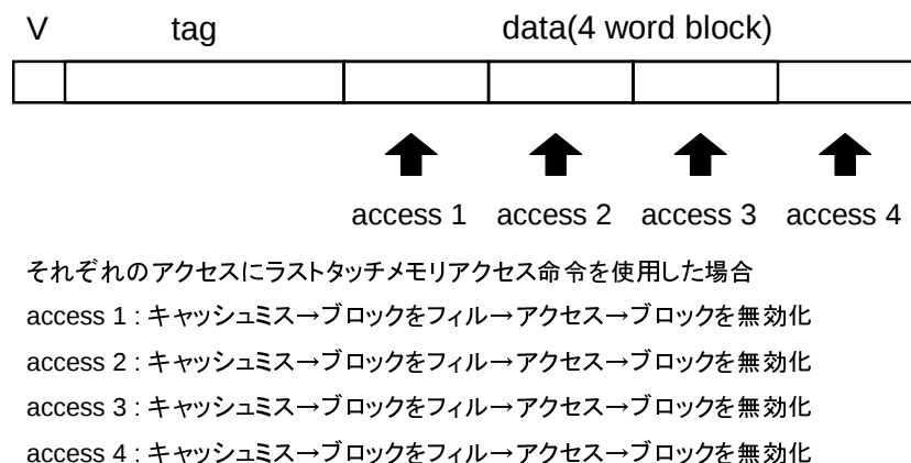
図 3.1: マルチワードブロックのキャッシュメモリでのラストタッチメモリアクセス命令
