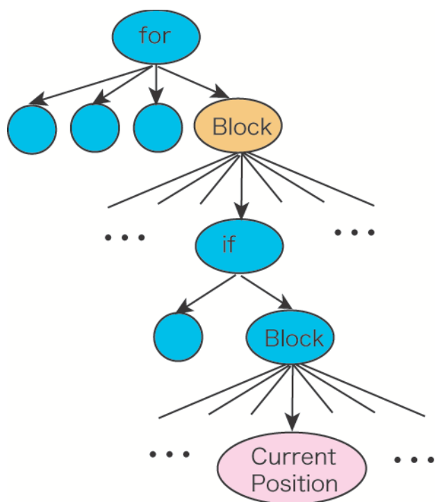
図 5.7: \text{depth}=1 , \text{des}=\text{FOR} のパラメータによる抽出
