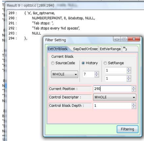
図 6.5: ツールの抽出結果 3
