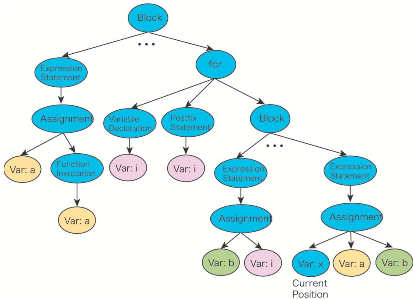
図 5.13: 表 5.4 の AST と、指定した代入文を追跡する様子
