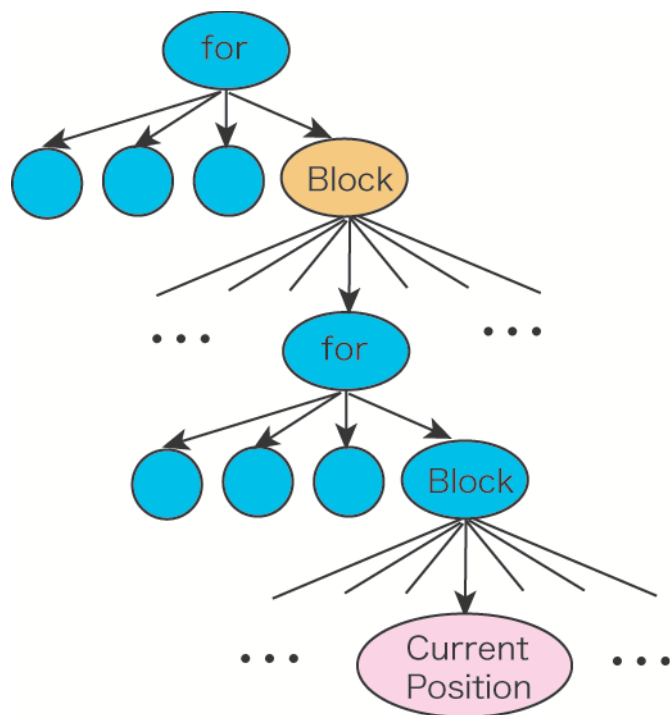
図 5.8: \text{pos}>0 , \text{depth}=2 , \text{des}=\text{FOR} のパラメータによる抽出
