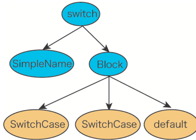
図 5.6: switch 文の AST の構造
