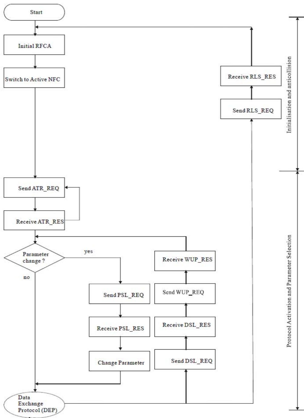
図 3.6: 受動モード時の有効化プロトコル
