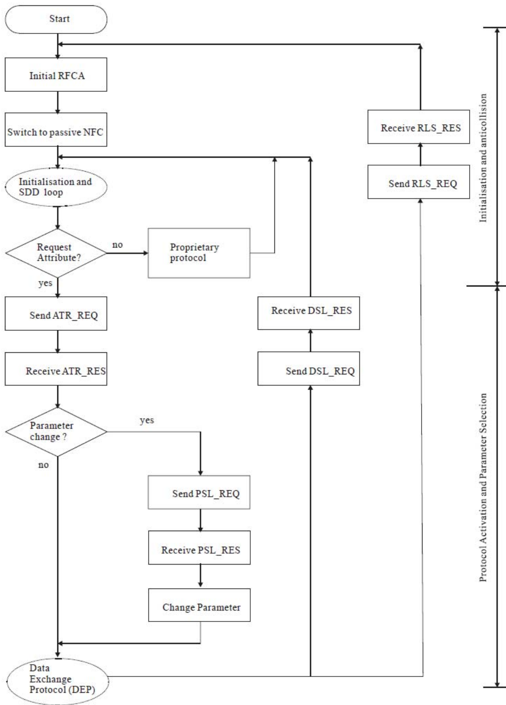
図 3.5: 受動モード時の有効化プロトコル
