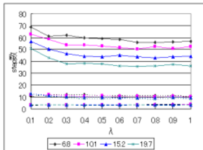
図 20 平均辺数 \bar{k} に対する Step 数
