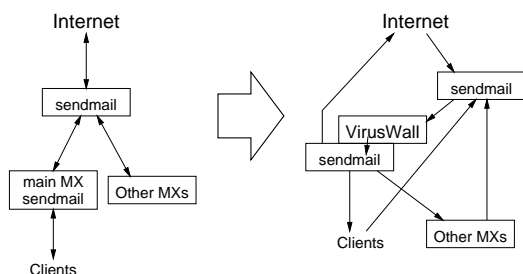
図 1 メールサーバの構成変更
