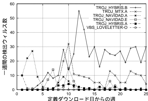
図4 定義日からの週ごとの検出ウイルス数 Fig.4 Weekly graph for major six viruses.
