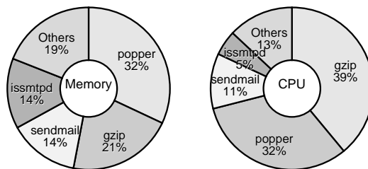
図5 ウィルス検査プロセスが占めるメモリとCPU時間の割合 Fig.5 Memory usage and CPU time of virus scan system.
