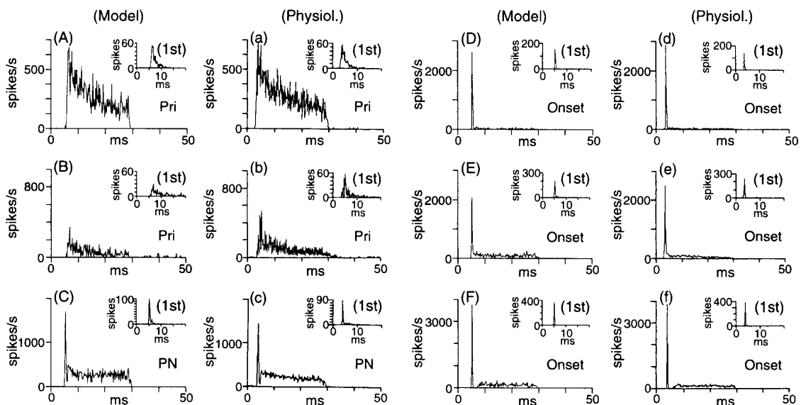
図-2 図-1の決定木により Pri 型, PN 型及び Onset 型に分類される応答の PST ヒストグラムと first spike latency ヒストグラム (Model): モデルの応答から作成。(Physiol.): 生理学的データ (Blackburn と Sachs, 1989)。(A), (B), (a), (b): Pri 型応答の PSTH。(C), (c): PN 型応答の PSTH。(D), (E), (F), (d), (e), (f): Onset 型応答の PSTH。(1st)に各応答型の first spike latency ヒストグラムを表示。First spike latency ヒストグラムにおける時間軸の縮尺は, PST ヒストグラムと同じ。
