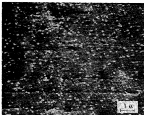
写真1. 粒状クロムT F SのSEM写真
