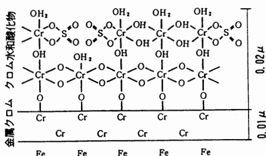
図3. T F S 皮膜構造の模式図
