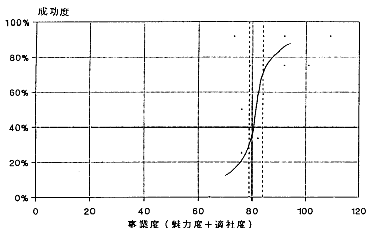
図5：成功確率曲線（事業年数5年以上14サンプル）
