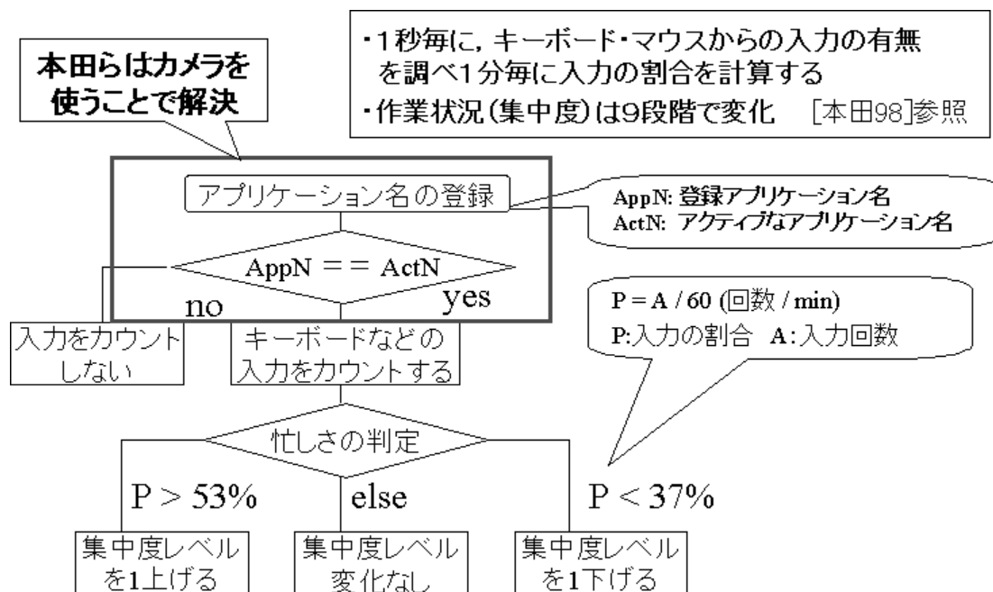
図 3.3 作業状況判定アルゴリズム
