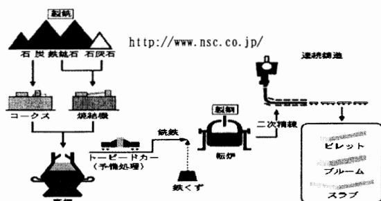
図1 一貫製鉄所の製造フロー
