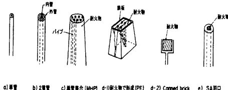
図4 羽口のバリエーション
