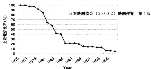
図3 上底吹転炉導入状況
