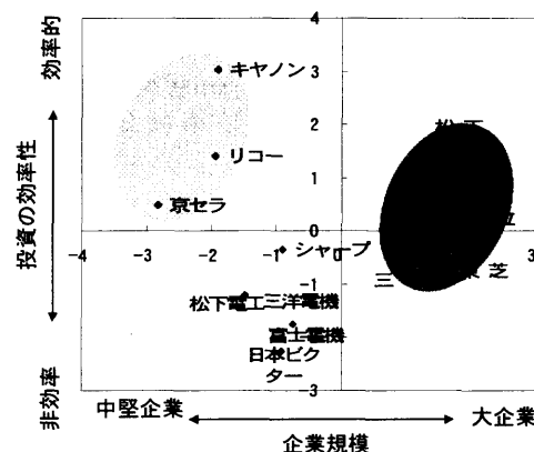
図7. 日本の代表的電気機械企業15社の主成分得点による散布図。
