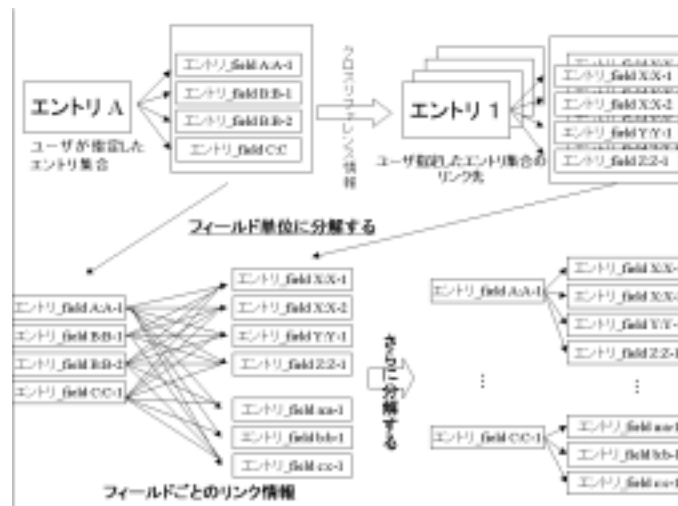
図 5.6: フィールド、フィールド間データ概念図
