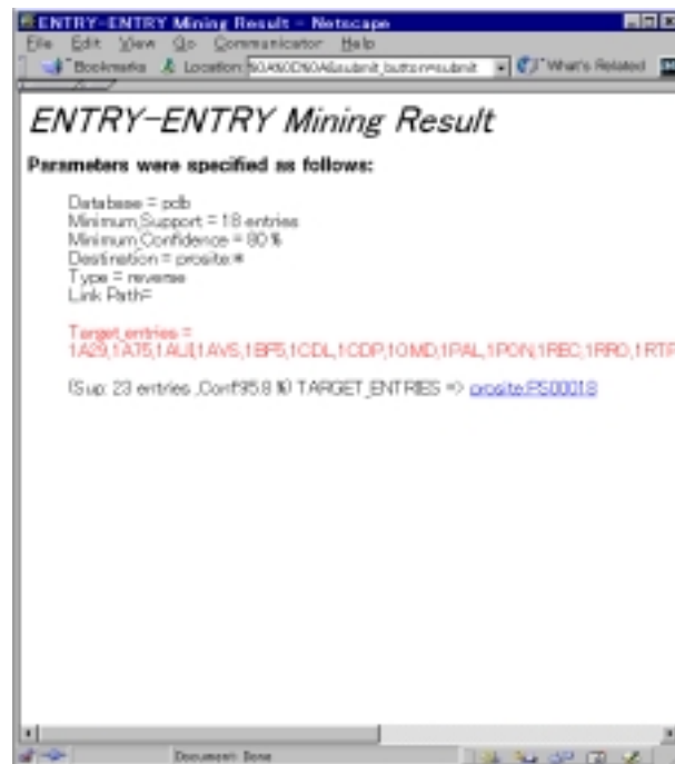
図 5.3: エントリ間データマイニングの計算結果 (ENTRY-ENTRY Data Mining)
