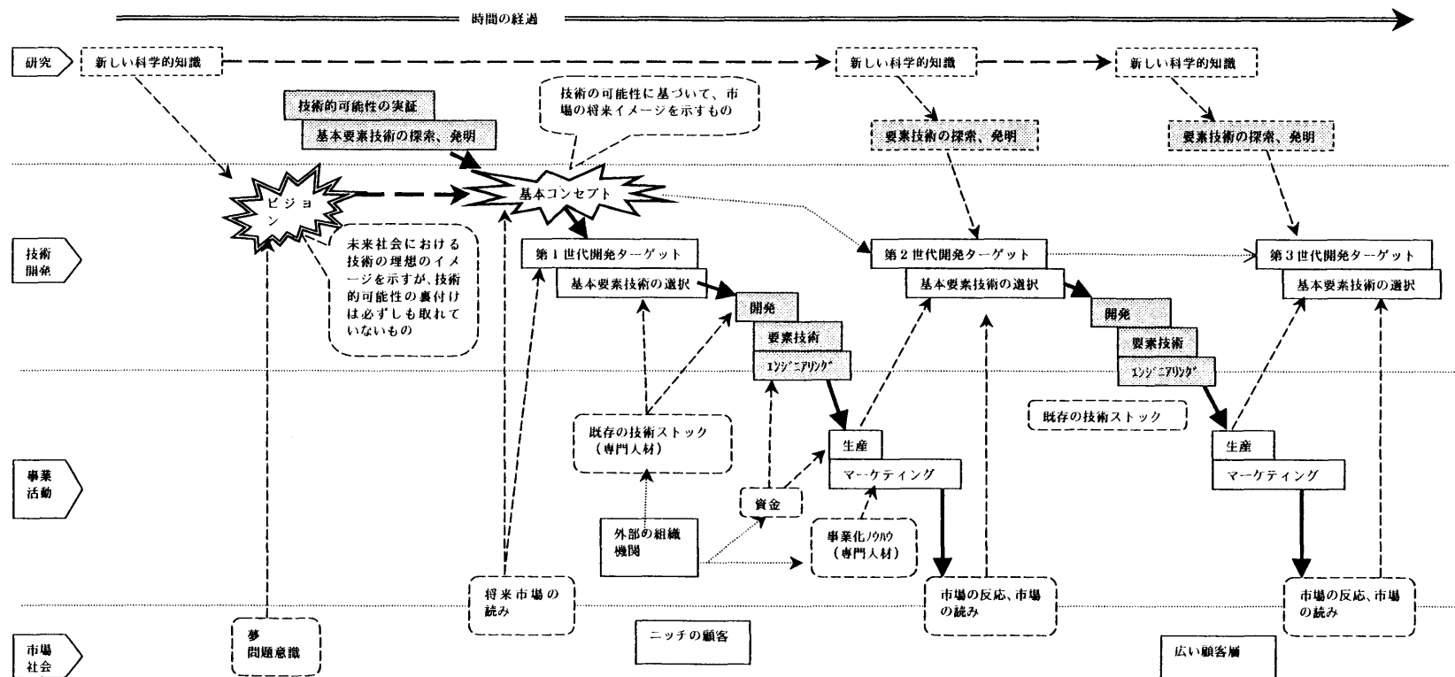
図表2 イノベーションのケーススタディとプロセス・モデルの仮説
