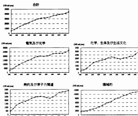
図3 ファインセラミックスの累積国内消費額の推移 (1981-2000) : 1995年価格基準
