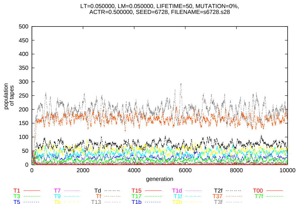
図 3.16: 例 2 における各テープの時系列 (ステップ = 3500 ~ 3700)
