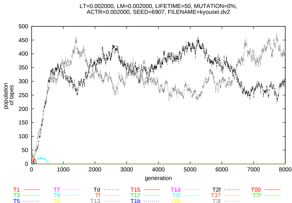
図 3.20: 例 4 における各テープの時系列
