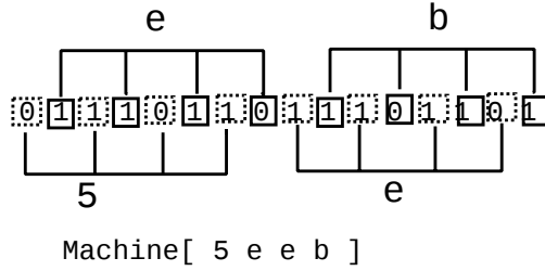
図 2.5: テープの翻訳
