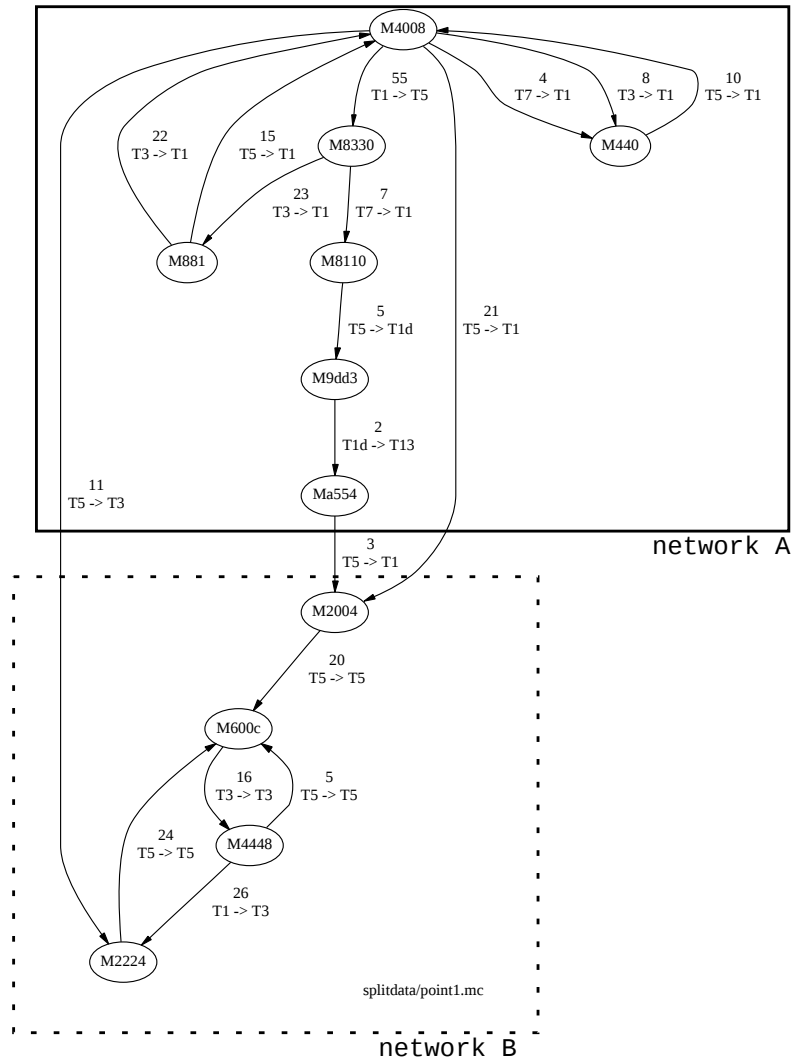
図 3.15: 例 1 における主なネットワーク (ステップ = 9000 ~ 9200)
