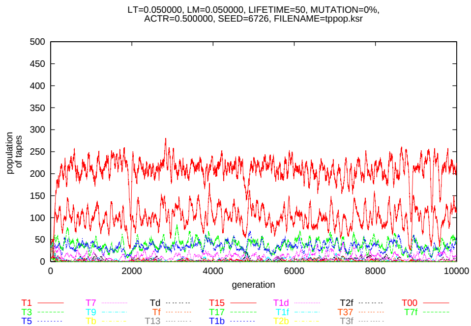
図 3.14: 例 1 における各テープの時系列
