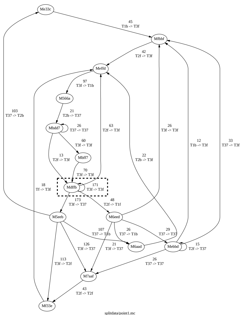
図 3.5: (T_{3f}, M_{dfbf}) による確率的自己複製の際の、主な反応のネットワーク
