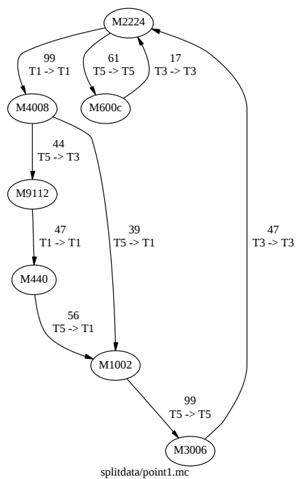
図 3.13: 図 3.11 の反応を構成する主要なネットワーク (ステップ = 3500 ~ 3700)
