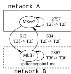
図 3.21: 例 4 におけるネットワーク (ステップ = 3500 ~ 4000)
