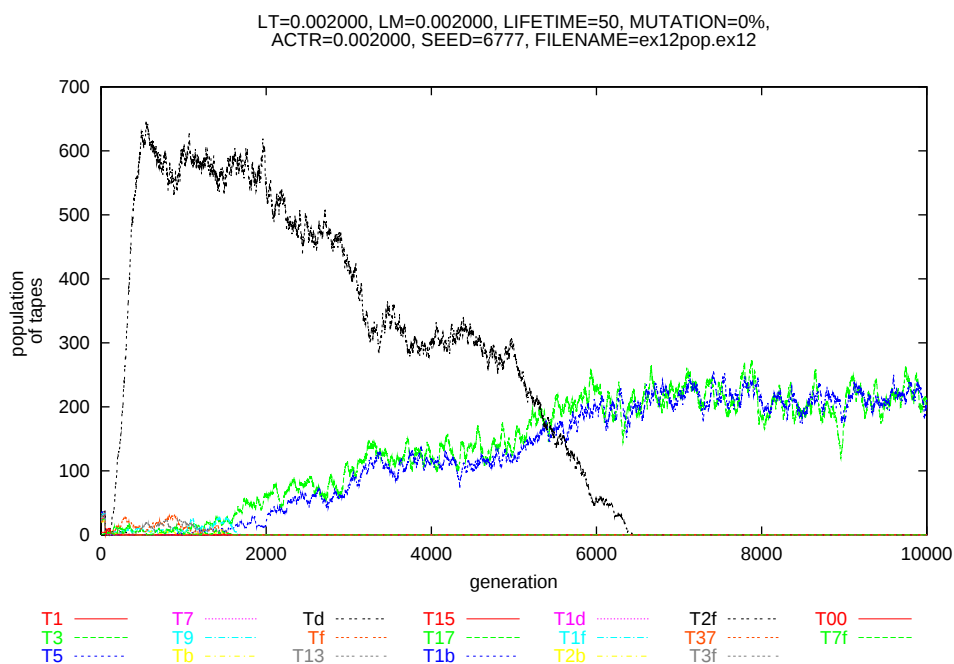
図 3.27: 例 6 における各テープの時系列
