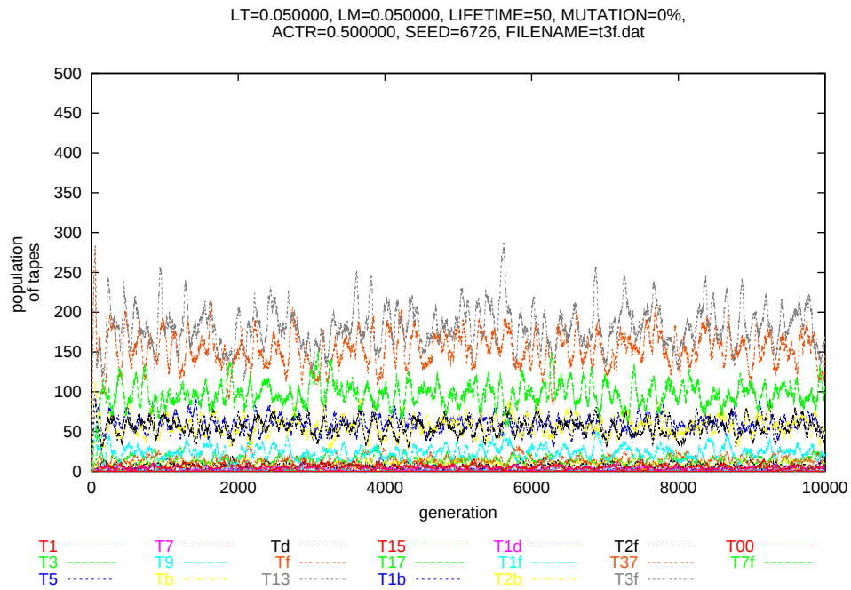
図 3.4: (T_{3f}, M_{dfb}) による確率的自己複製の際の，各テープの時系列グラフ
