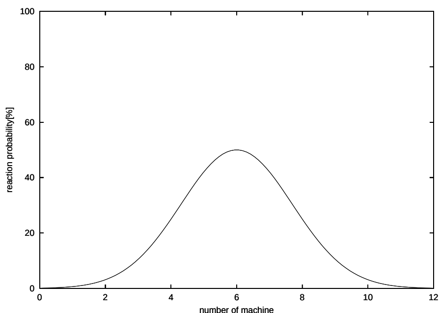
図 2.6: 局所的資源制約における，反応確率，及び半径 r_g 内の他のマシンの個数との関係
