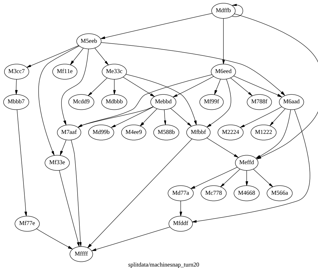
図 3.9: 初期状態として 50 個ずつの T_{3f} , M_{df\,fb} を配置したときのネットワークの発展 (ステップ = 20)
