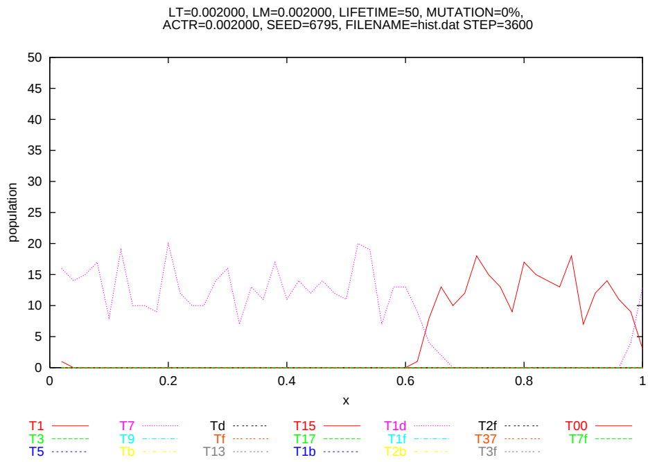
図 3.19: 例 3 における各位置での各タイプのヒストグラム (ステップ = 3600)
