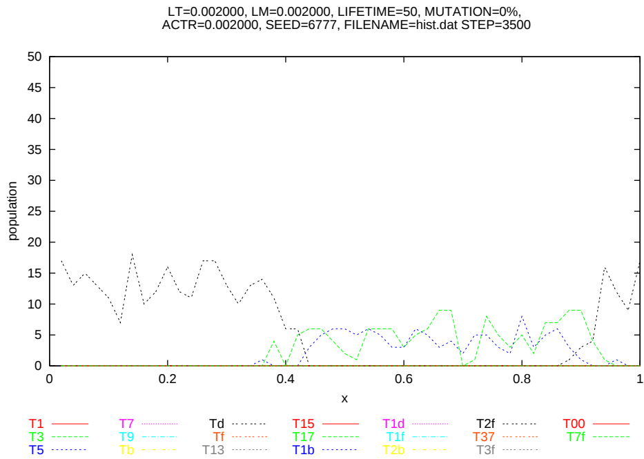
図 3.29: 例 6 における各タイプのヒストグラム (ステップ = 3500)
