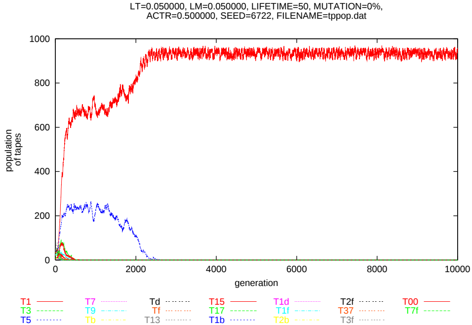
図 3.1: (T_1, M_{1002}) による自己複製の際の，各テープの時系列グラフ
