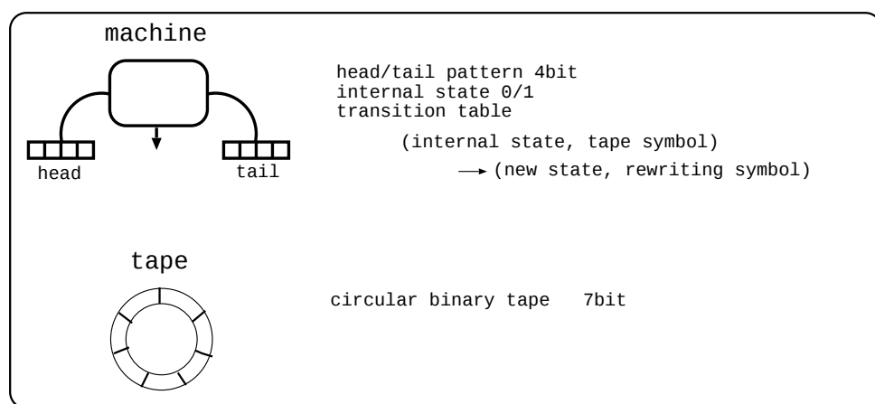
図 2.1: テープ, マシンの模式図
