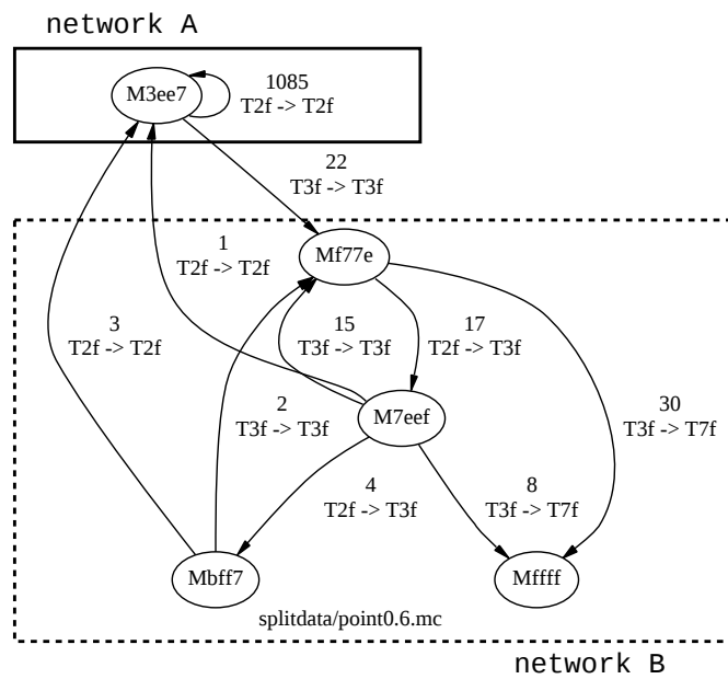
図 3.25: 例 5 におけるネットワーク (ステップ = 3500 ~ 4000) ネットワーク B がある場合
