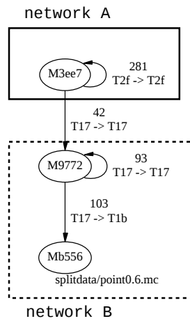
図 3.28: 例 6 における主なネットワーク (ステップ = 3500 ~ 4000)
