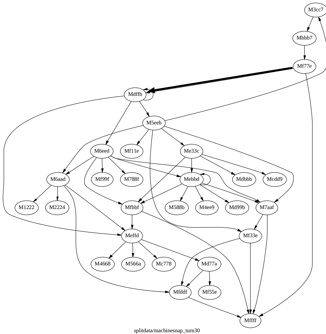
図 3.10: 初期状態として 50 個ずつの T_{3f} , M_{dfb} を配置したときのネットワークの発展 (ステップ = 30)
