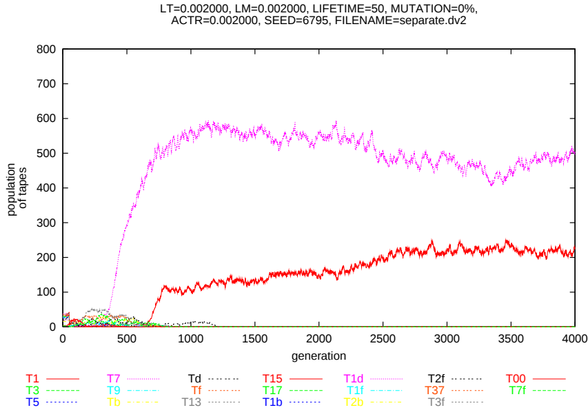
図 3.18: 例 3 における各テープの時系列
