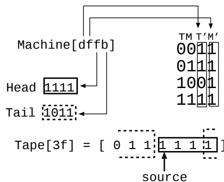
図 2.3: マシンのヘッド, テール, 遷移表との対応, 及びテープ上の探索 遷移表の上部 T,M の列は現在の状態, T',M' の列は遷移後の状態を表す
