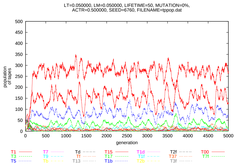
図 3.11: 観察されたコアネットワークにおける各テープ時系列
