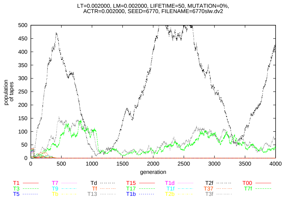
図 3.23: 例 5 における各テープの時系列
